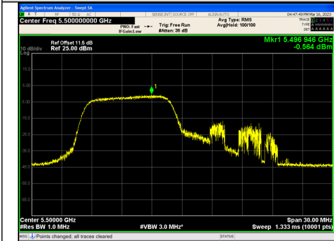
IEEE 802.11ax_Channel 100_20MHz_Antenna 2_RU&Index 52RU37
