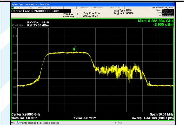
IEEE 802.11ax_Channel 52_20MHz_Antenna 1_RU&Index 52RU37
