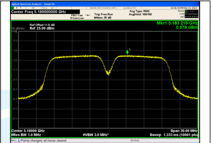
IEEE 802.11ax_Channel 36_20MHz_Antenna 1_RU&Index 106RU53
