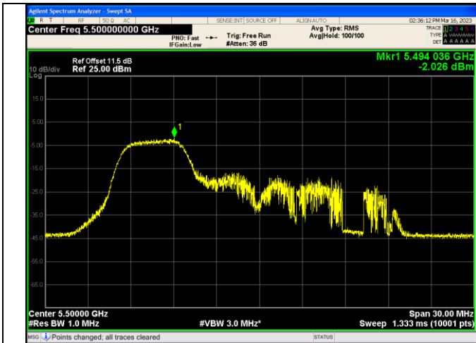
IEEE 802.11ax_Channel 100_20MHz_Antenna 2_RU&Index 26RU0
