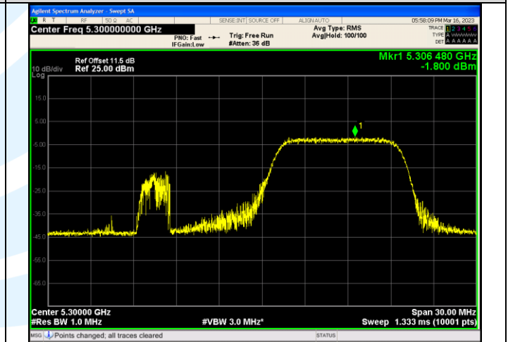
IEEE 802.11ax_Channel 60_20MHz_Antenna 3_RU&Index 52RU39
