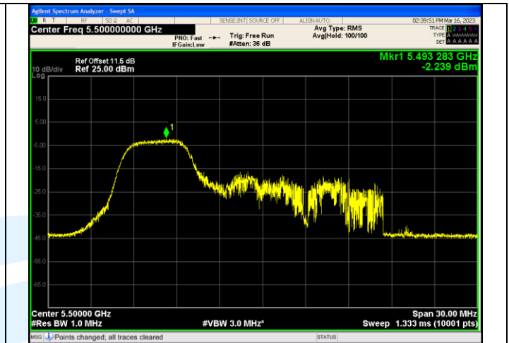
IEEE 802.11ax_Channel 100_20MHz_Antenna 3_RU&Index 26RU0
