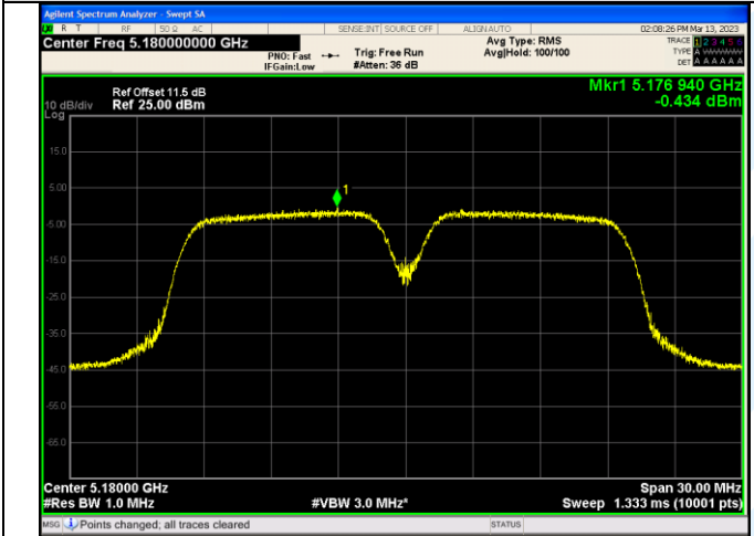
IEEE 802.11ax_Channel 36_20MHz_Antenna 2_RU&Index 106RU53
