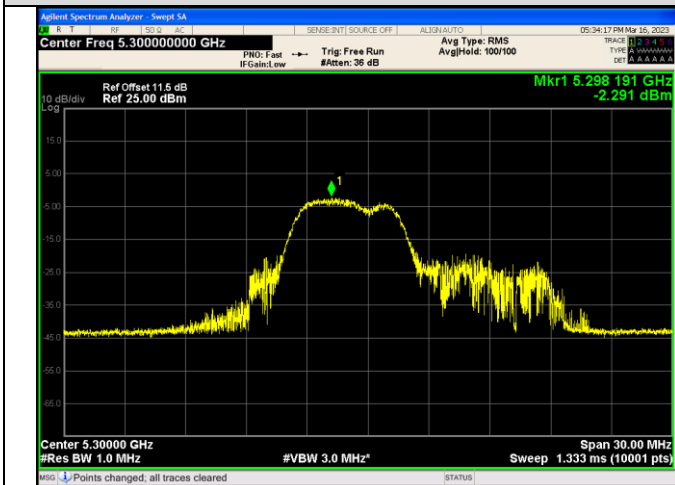
IEEE 802.11ax_Channel 60_20MHz_Antenna 0_RU&Index 26RU4
