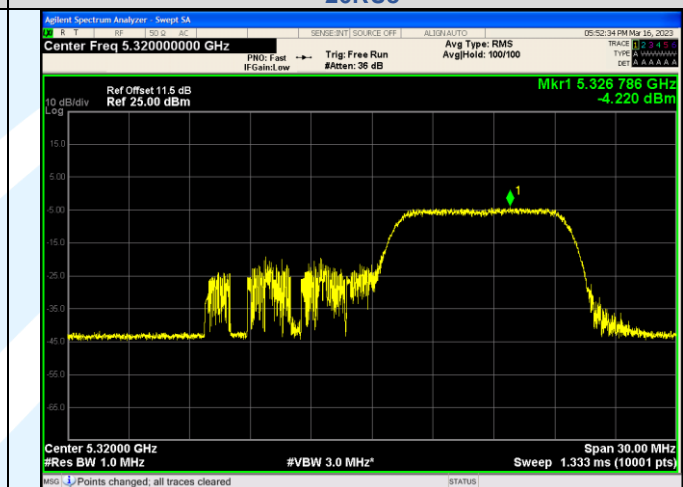
IEEE 802.11ax_Channel 64_20MHz_Antenna 1_RU&Index 52RU40
