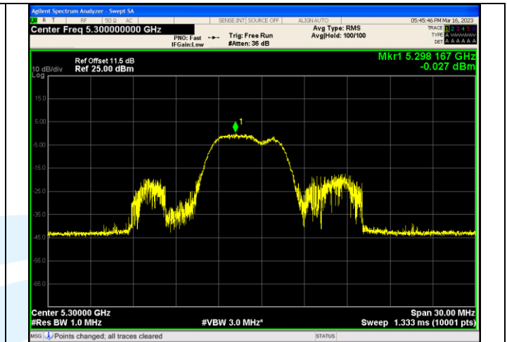
IEEE 802.11ax_Channel 60_20MHz_Antenna 3_RU&Index 26RU4
