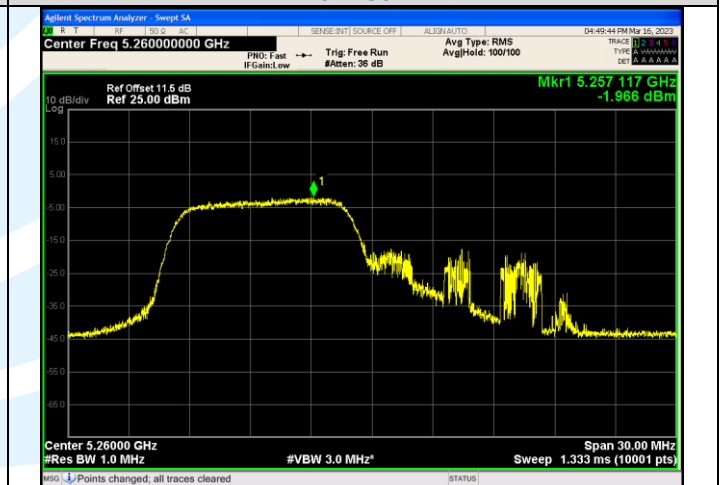
IEEE 802.11ax_Channel 52_20MHz_Antenna 3_RU&Index 52RU37
