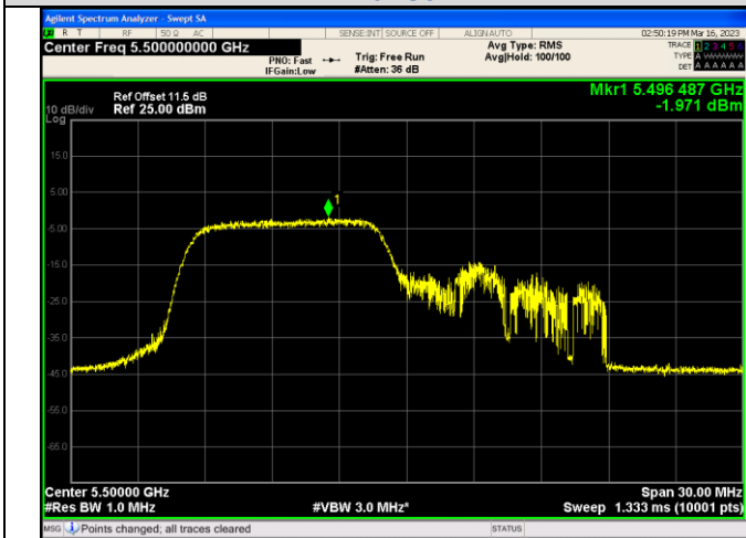
IEEE 802.11ax_Channel 100_20MHz_Antenna 0_RU&Index 52RU37
