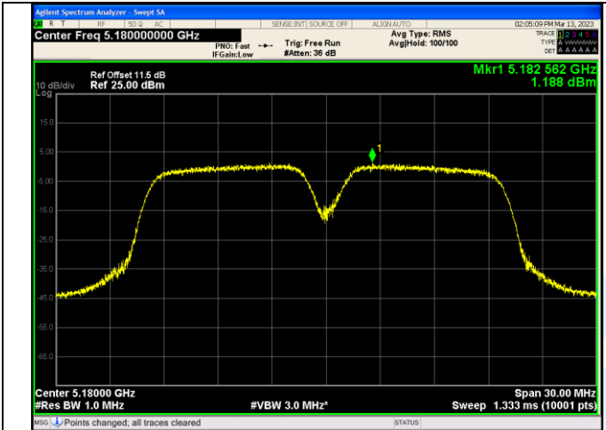
IEEE 802.11ax_Channel 36_20MHz_Antenna 0_RU&Index 106RU53
