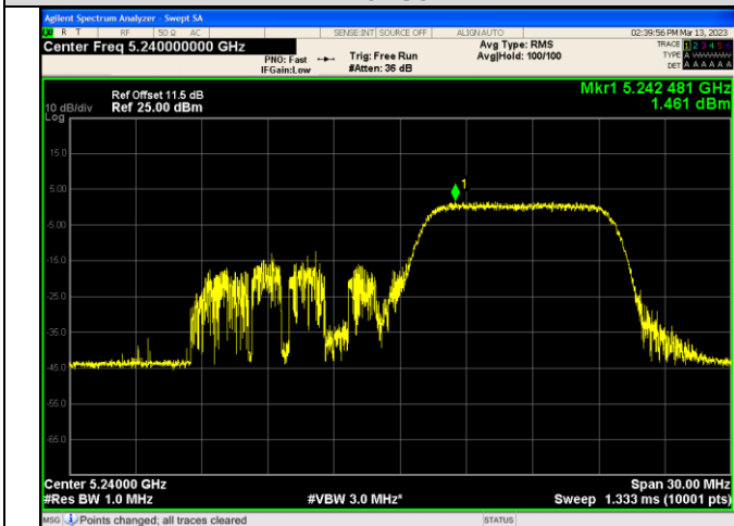
IEEE 802.11ax_Channel 48_20MHz_Antenna 0_RU&Index 52RU40
