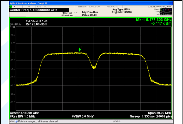
IEEE 802.11ax_Channel 36_20MHz_Antenna 3_RU&Index 106RU53
