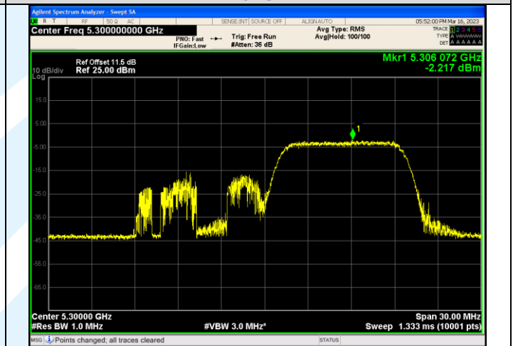
IEEE 802.11ax_Channel 60_20MHz_Antenna 1_RU&Index 52RU39
