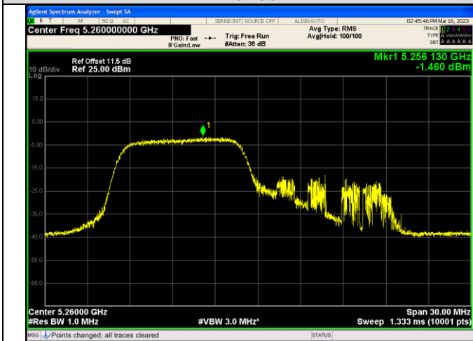
IEEE 802.11ax_Channel 52_20MHz_Antenna 0_RU&Index 52RU37
