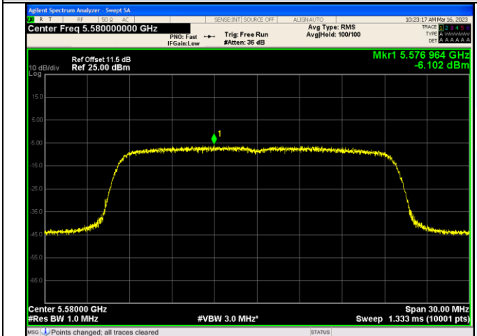
IEEE 802.11ax_Channel 116_20MHz_Antenna 3_RU&Index SU
