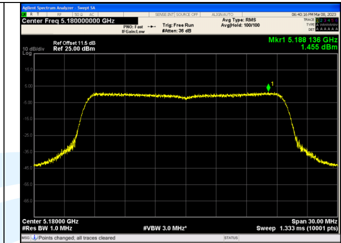
IEEE 802.11ax_Channel 36_20MHz_Antenna 3_RU&Index SU
