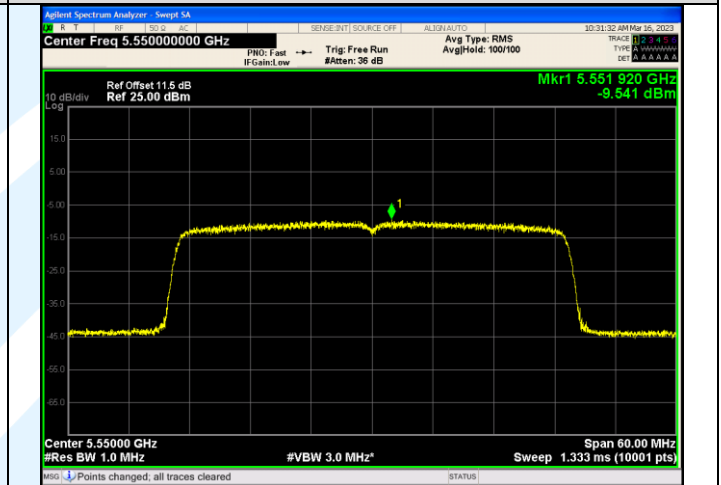
IEEE 802.11ax_Channel 110_40MHz_Antenna 3_RU&Index SU
