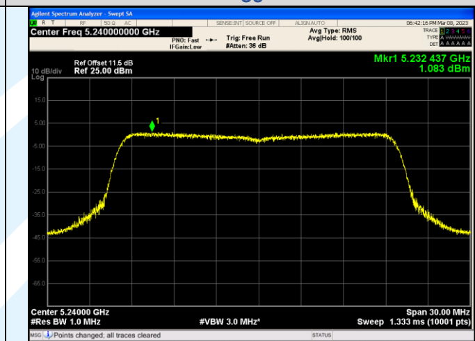
IEEE 802.11ax_Channel 48_20MHz_Antenna 3_RU&Index SU
