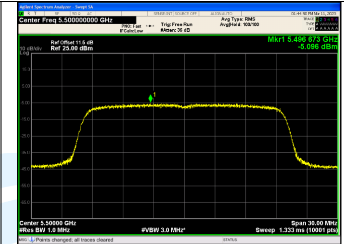
IEEE 802.11ax_Channel 100_20MHz_Antenna 3_RU&Index SU
