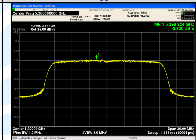
IEEE 802.11ax_Channel 60_20MHz_Antenna 3_RU&Index SU
