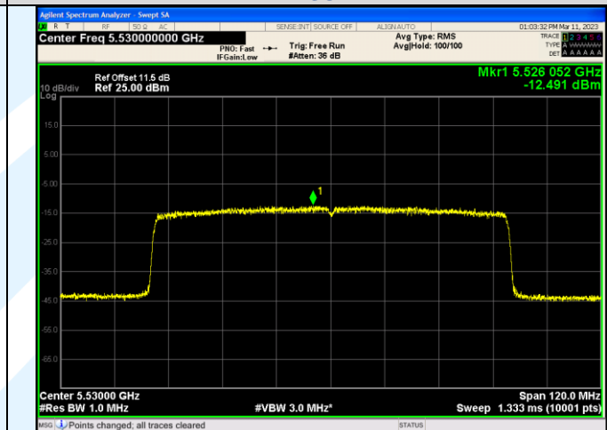
IEEE 802.11ax_Channel 106_80MHz_Antenna 2_RU&Index SU
