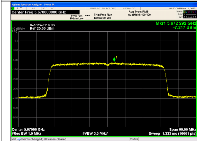
IEEE 802.11ax_Channel 134_40MHz_Antenna 3_RU&Index SU
