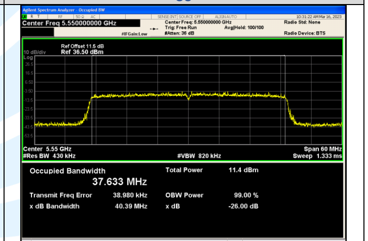
IEEE 802.11ax_Channel 110_40MHz_Antenna 3_RU&Index SU
