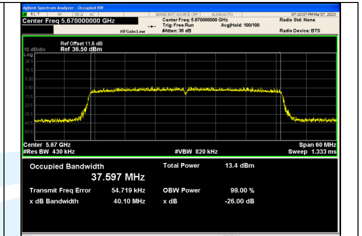
IEEE 802.11ax_Channel 134_40MHz_Antenna 1_RU&Index SU
