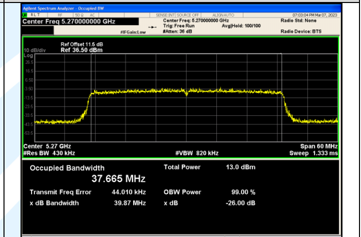
IEEE 802.11ax_Channel 54_40MHz_Antenna 1_RU&Index SU
