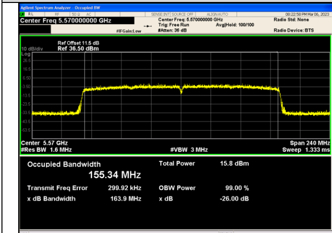
IEEE 802.11ax_Channel 114_160MHz_Antenna 0_RU&Index SU
