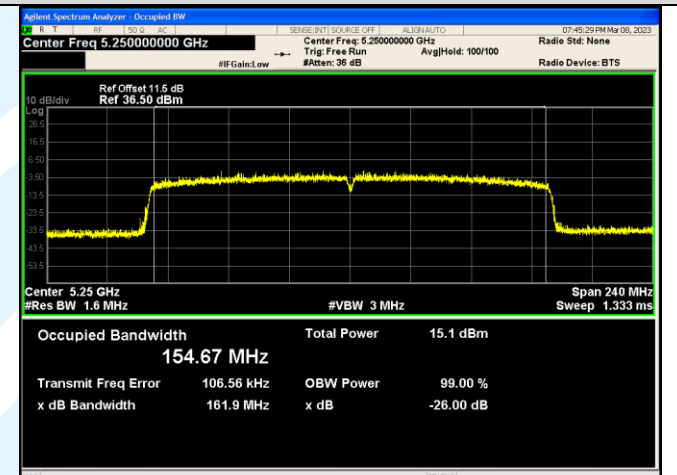
IEEE 802.11ax_Channel 50_160MHz_Antenna 3_RU&Index SU
