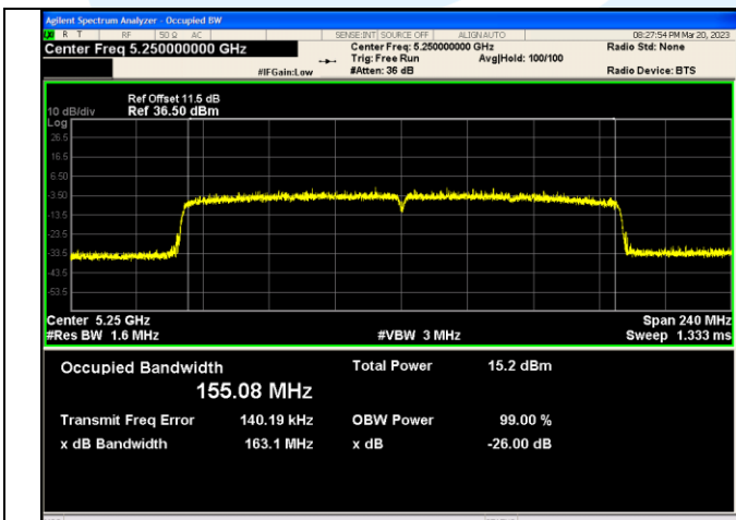
IEEE 802.11ax_Channel 50_80+80MHz_Antenna 0_RU&Index SU
