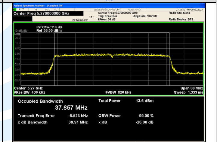
IEEE 802.11ax_Channel 54_40MHz_Antenna 3_RU&Index SU
