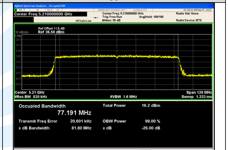
IEEE 802.11ax_Channel 42_80MHz_Antenna 1_RU&Index SU
