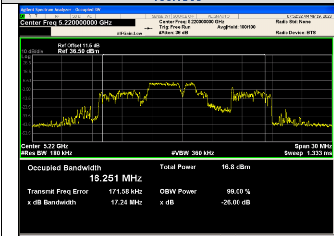
IEEE 802.11ax_Channel 44_20MHz_Antenna 0_RU&Index 26RU4
