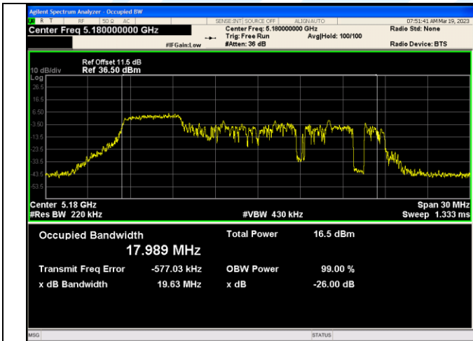
IEEE 802.11ax_Channel 36_20MHz_Antenna 0_RU&Index 26RU0
