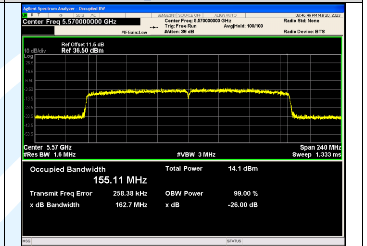
IEEE 802.11ax_Channel 114_80+80MHz_Antenna 1_RU&Index SU
