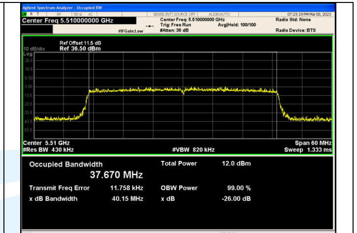
IEEE 802.11ax_Channel 102_40MHz_Antenna 3_RU&Index SU
