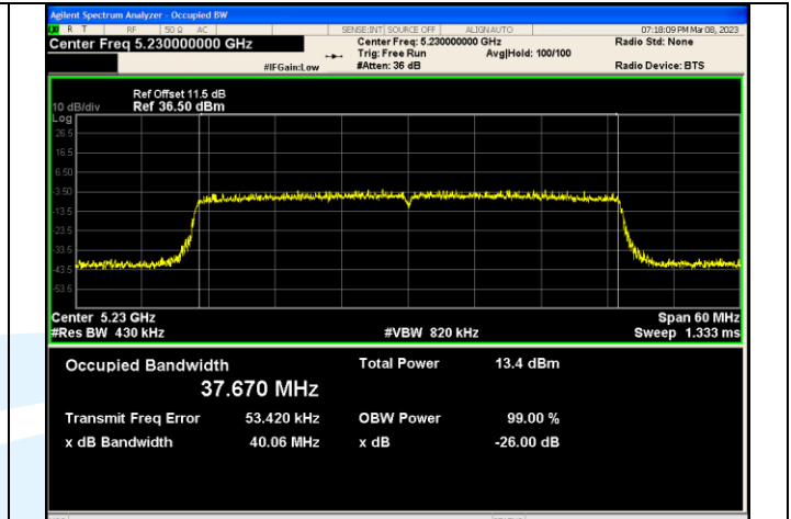
IEEE 802.11ax_Channel 46_40MHz_Antenna 3_RU&Index SU
