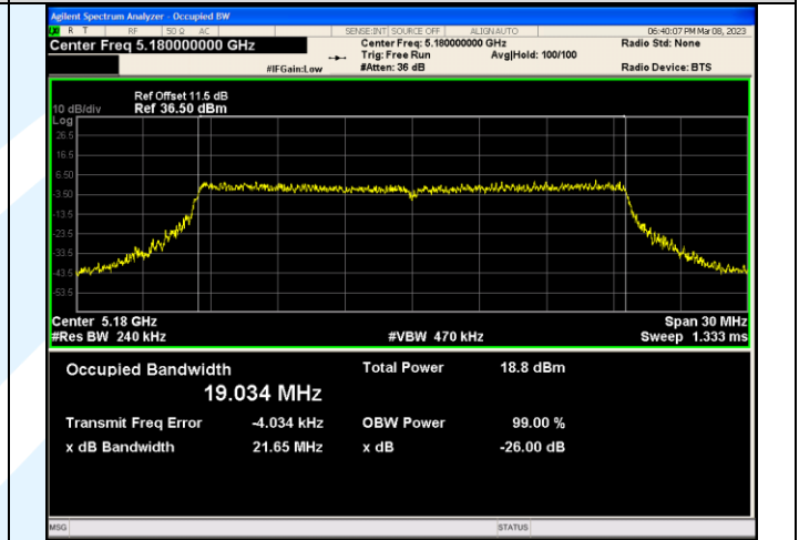
IEEE 802.11ax_Channel 36_20MHz_Antenna 3_RU&Index SU
