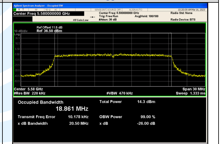
IEEE 802.11ax_Channel 116_20MHz_Antenna 1_RU&Index SU
