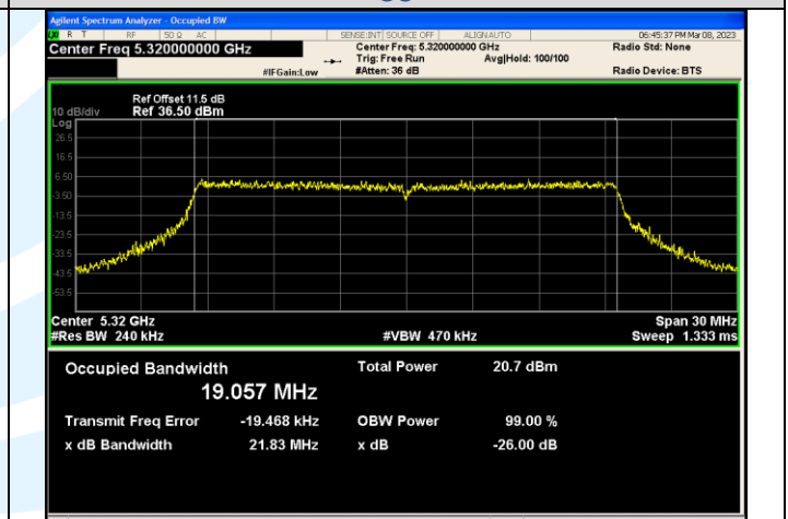
IEEE 802.11ax_Channel 64_20MHz_Antenna 3_RU&Index SU
