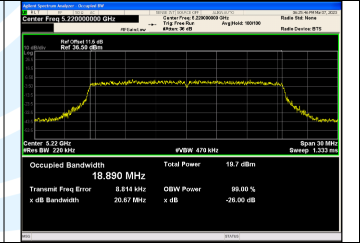
IEEE 802.11ax_Channel 44_20MHz_Antenna 1_RU&Index SU
