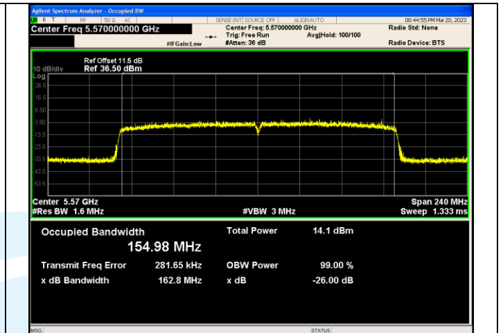
IEEE 802.11ac_Channel 114_80+80MHz_Antenna 1
