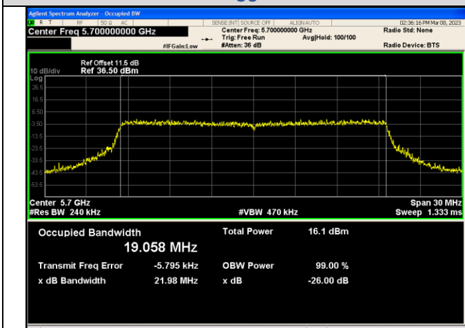
IEEE 802.11ax_Channel 140_20MHz_Antenna 2_RU&Index SU
