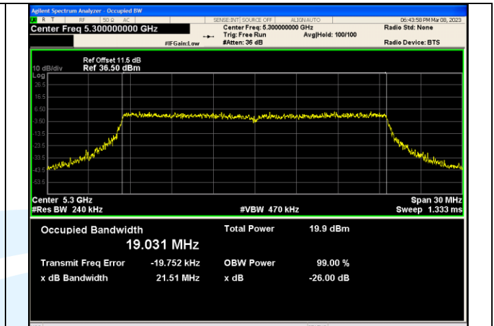
IEEE 802.11ax_Channel 60_20MHz_Antenna 3_RU&Index SU
