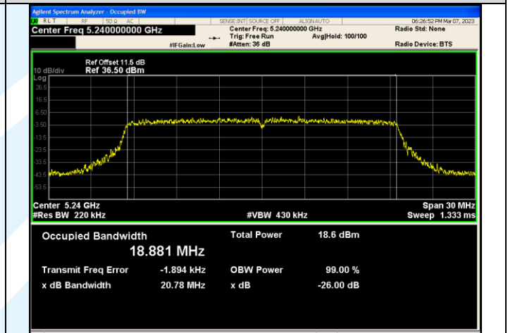
IEEE 802.11ax_Channel 48_20MHz_Antenna 1_RU&Index SU
