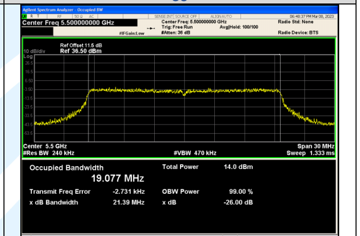
IEEE 802.11ax_Channel 100_20MHz_Antenna 3_RU&Index SU
