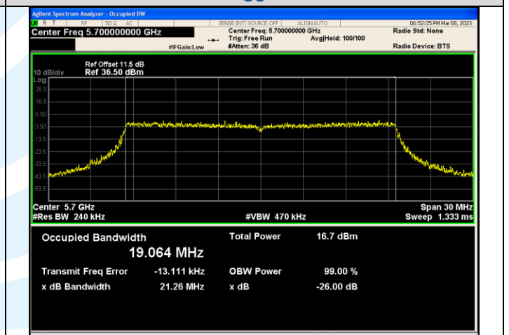
IEEE 802.11ax_Channel 140_20MHz_Antenna 3_RU&Index SU
