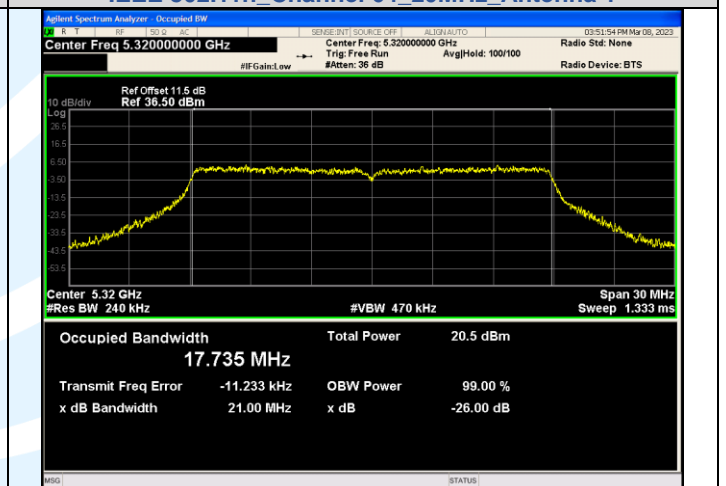
IEEE 802.11n_Channel 64_20MHz_Antenna 3
