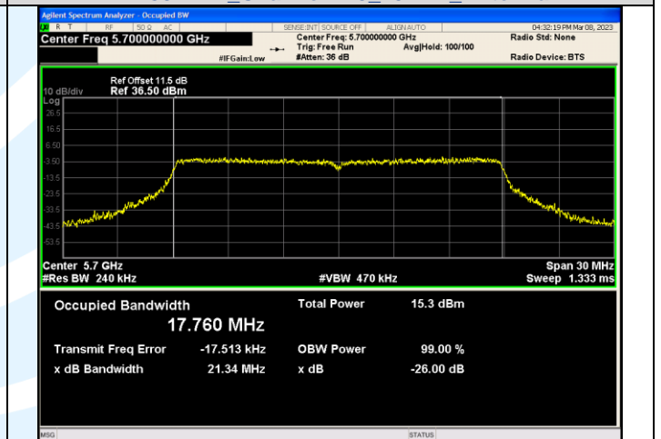
IEEE 802.11n_Channel 140_20MHz_Antenna 3
