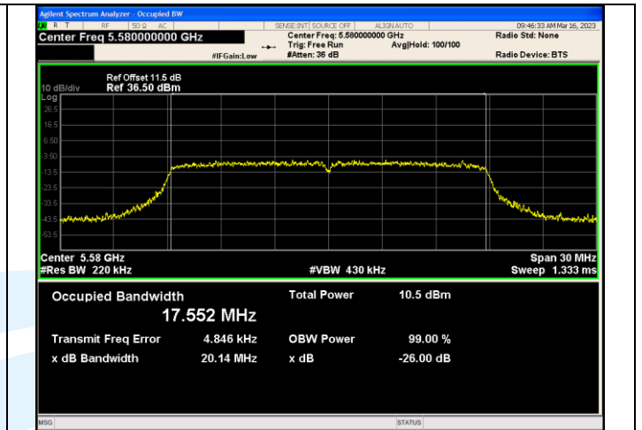
IEEE 802.11n_Channel 116_20MHz_Antenna 3
