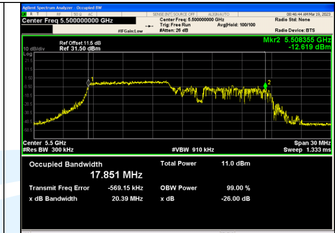
IEEE 802.11ax_Channel 100_20MHz_Antenna 1_RU&Index 52RU37
