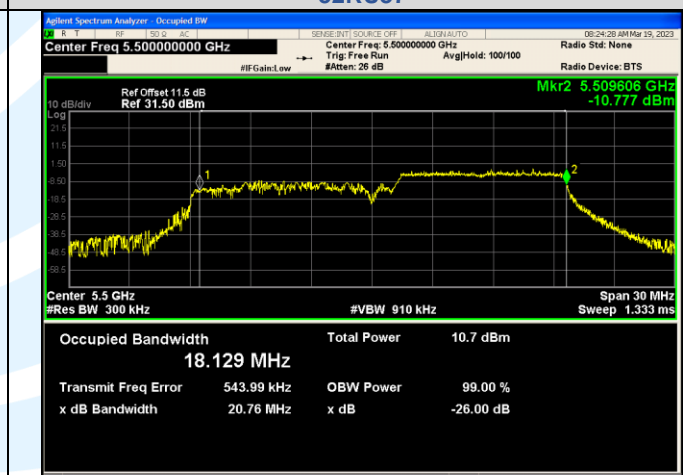
IEEE 802.11ax_Channel 100_20MHz_Antenna 1_RU&Index 106RU53
