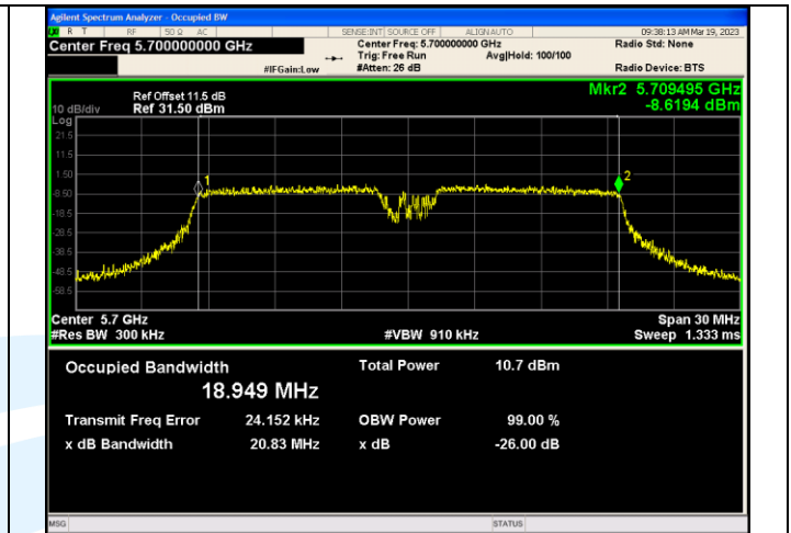
IEEE 802.11ax_Channel 140_20MHz_Antenna 3_RU&Index 106RU53
