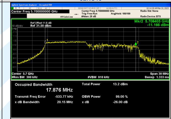
IEEE 802.11ax_Channel 140_20MHz_Antenna 3_RU&Index 52RU40
