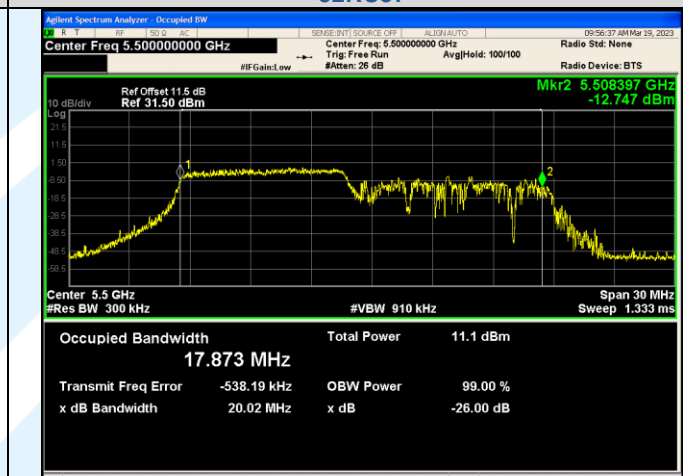
IEEE 802.11ax_Channel 100_20MHz_Antenna 3_RU&Index 52RU37
