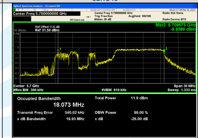
IEEE 802.11ax_Channel 140_20MHz_Antenna 1_RU&Index 106RU53
