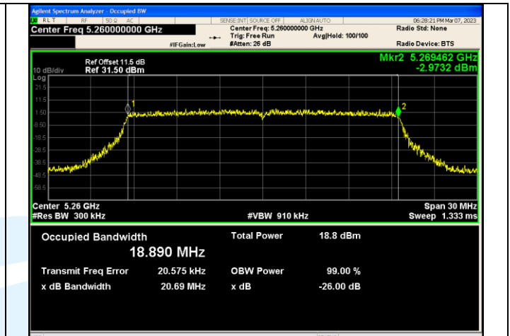
IEEE 802.11ax_Channel 52_20MHz_Antenna 1_RU&Index SU
