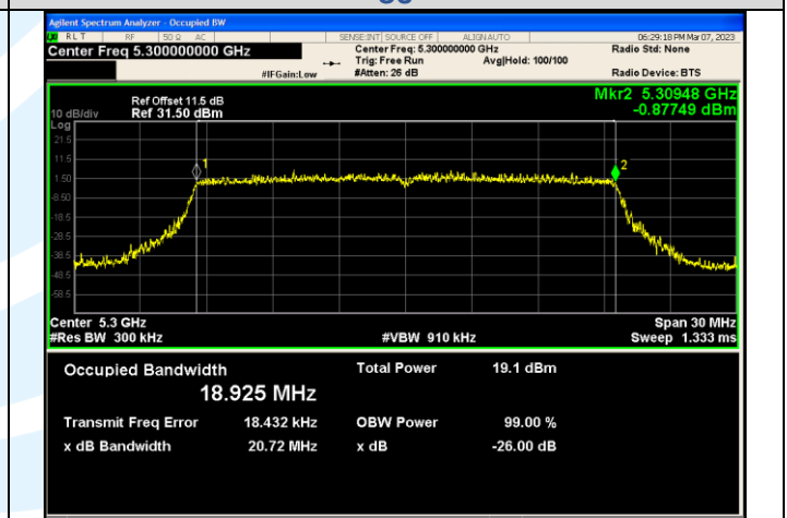
IEEE 802.11ax_Channel 60_20MHz_Antenna 1_RU&Index SU
