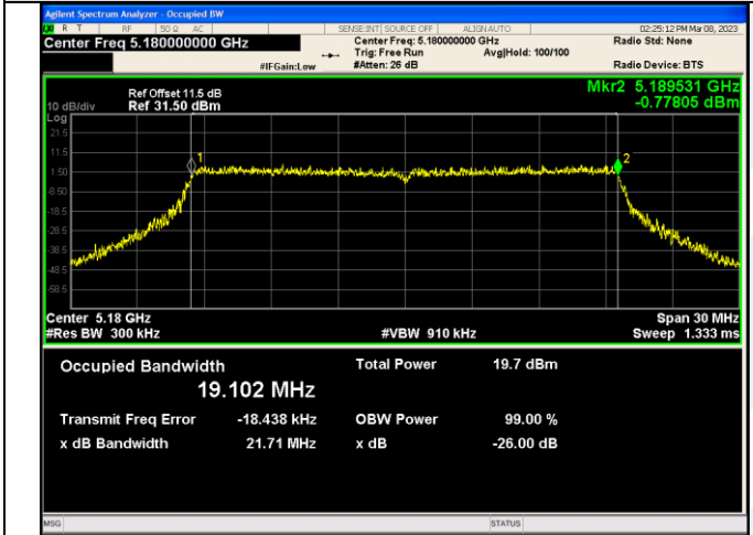
IEEE 802.11ax_Channel 36_20MHz_Antenna 2_RU&Index SU
