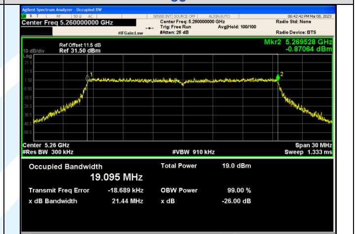
IEEE 802.11ax_Channel 52_20MHz_Antenna 3_RU&Index SU
