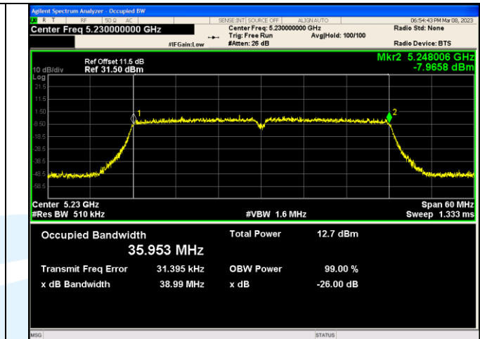
IEEE 802.11n_Channel 46_40MHz_Antenna 3
