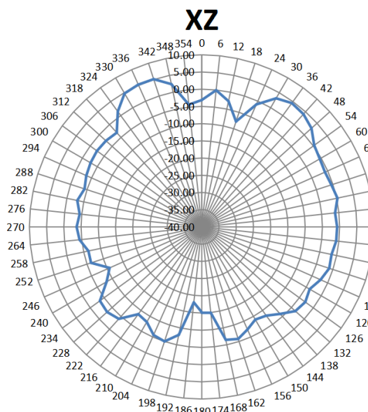
5G 辐射方向图 Radiation Patterns (unit: dB) 5G 5650MHz
