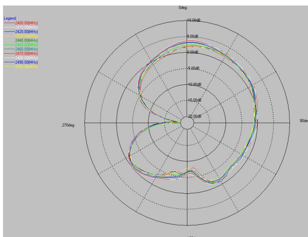
2.4G phi=0deg
