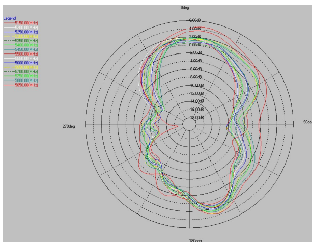
5G theta=90deg
