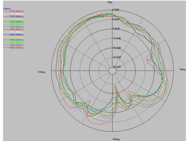
5G phi=90deg
