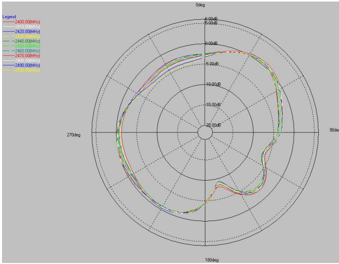
2.4G theta=90deg
