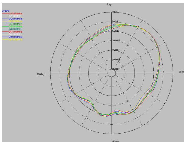
2.4G phi=0deg
