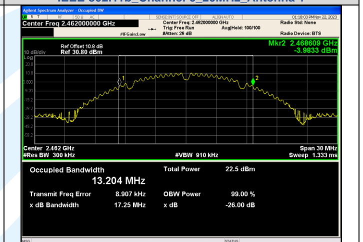
IEEE 802.11b_Channel 11_20MHz_Antenna 1
