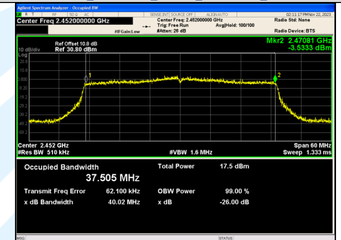
IEEE 802.11ax Channel 9 40MHz Antenna 1_RU&Index SU
