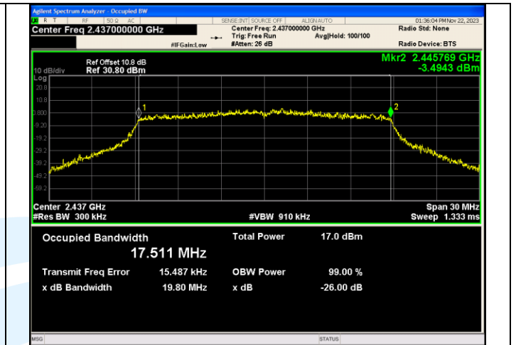
IEEE 802.11n_Channel 6_20MHz_Antenna 1
