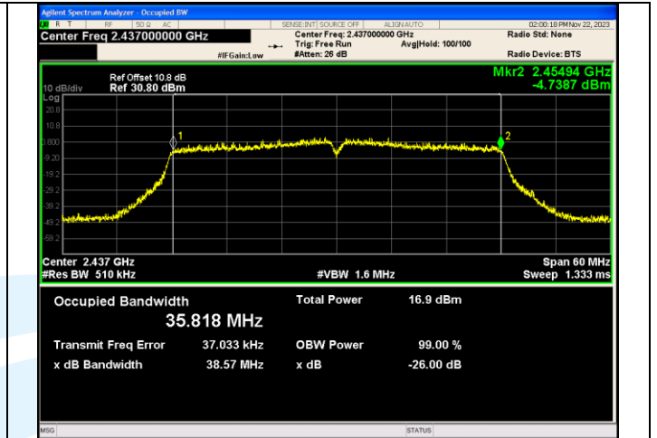
IEEE 802.11n_Channel 6_40MHz_Antenna 1
