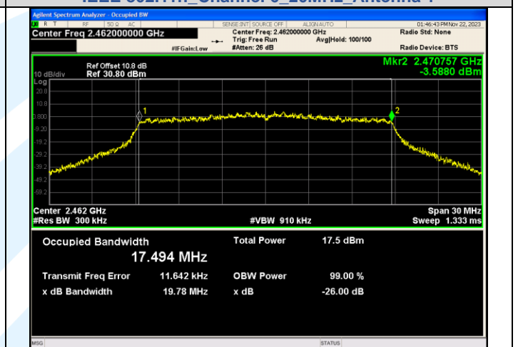
IEEE 802.11n_Channel 11_20MHz_Antenna 1
