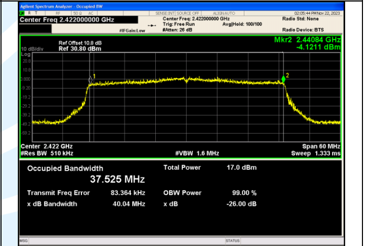
IEEE 802.11ax_Channel 3_40MHz_Antenna 1_RU&Index SU
