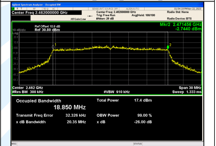
IEEE 802.11ax_Channel 11_20MHz_Antenna 1_RU&Index SU
