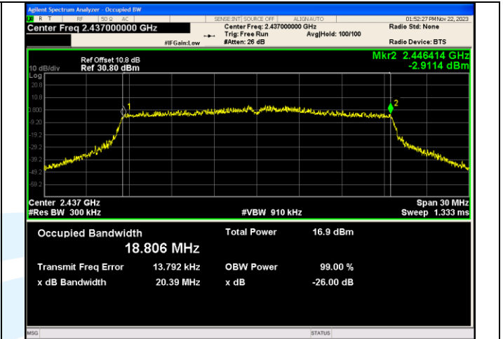
IEEE 802.11ax_Channel 6_20MHz_Antenna 1_RU&Index SU
