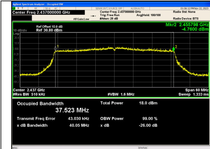
IEEE 802.11ax Channel 6 40MHz Antenna 0_RU&Index SU
