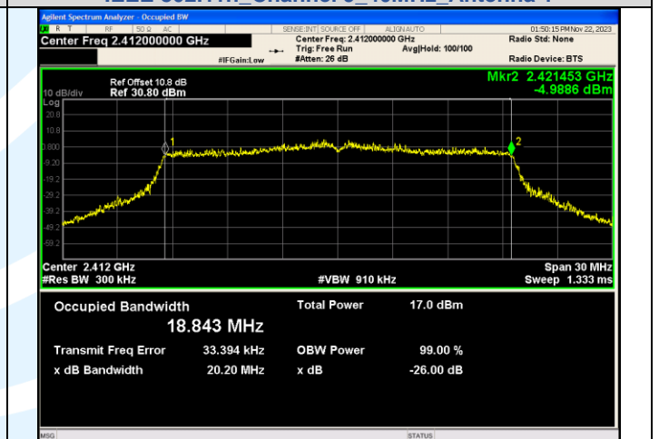
IEEE 802.11ax_Channel 1_20MHz_Antenna 1_RU&Index SU
