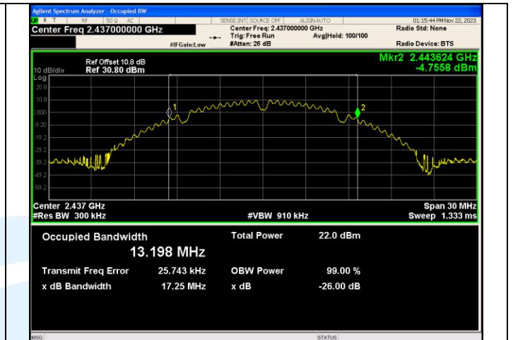
IEEE 802.11b_Channel 6_20MHz_Antenna 1
