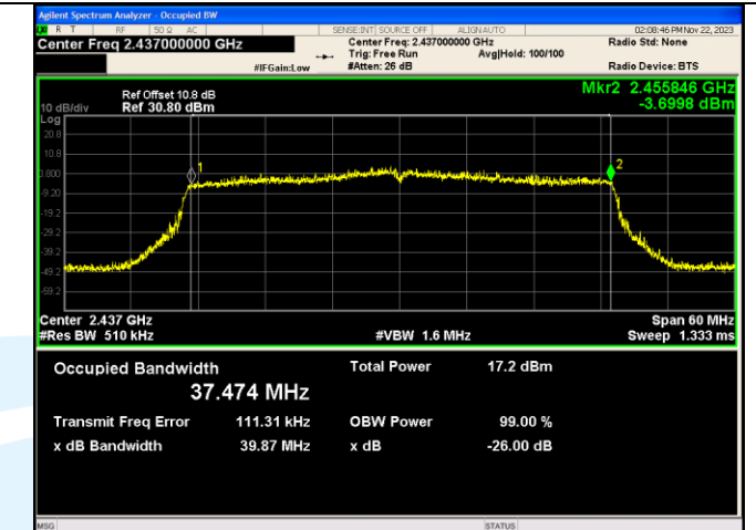
IEEE 802.11ax Channel 6 40MHz Antenna 1_RU&Index SU
