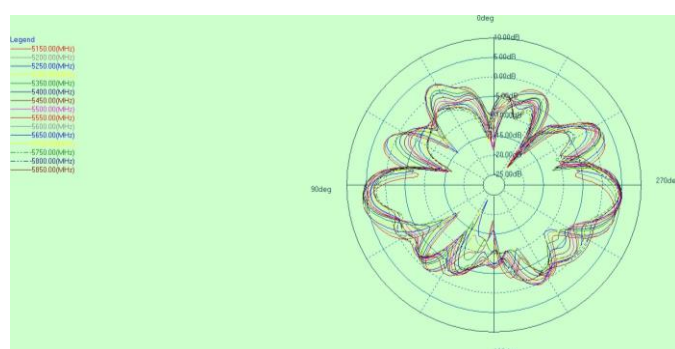
phi=0deg
