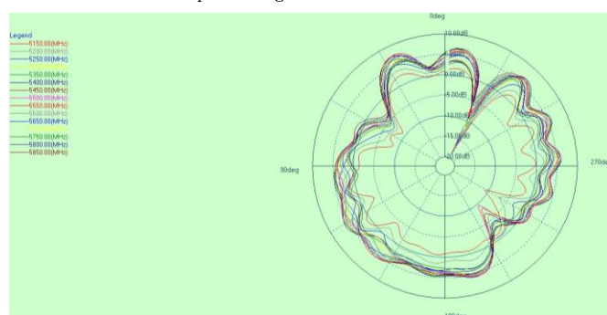
theta=90deg
