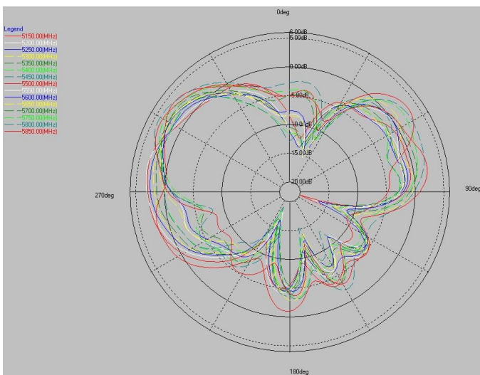
5G theta=90deg
