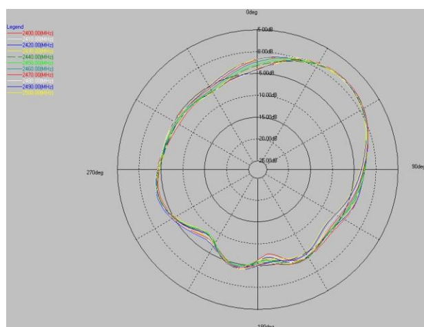
2.4G phi=0deg
