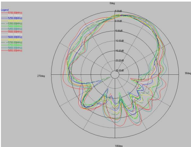
5G phi=0deg
