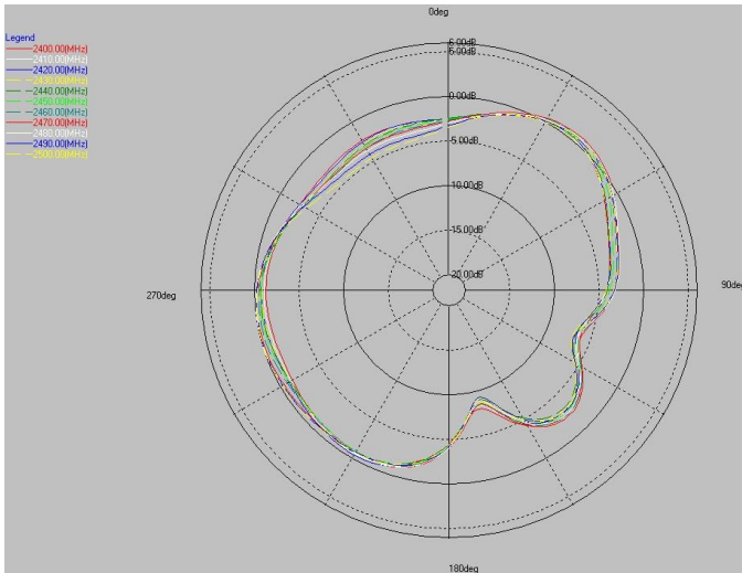
2.4G theta=90deg
