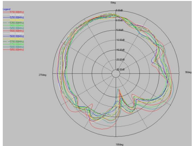
5G phi=90deg
