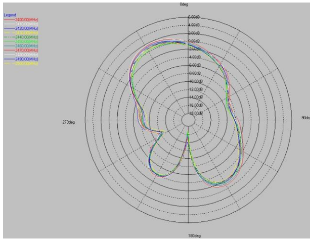
2.4G theta=90deg
