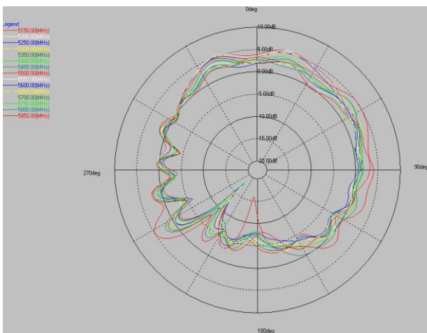
5G phi=0deg
