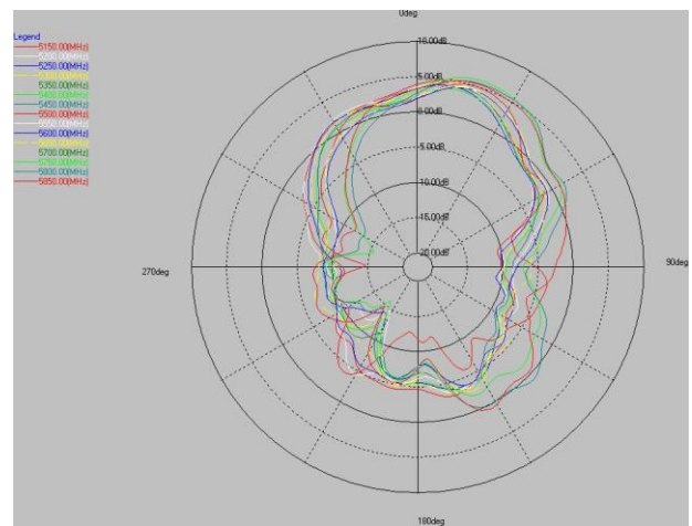
5G phi=90deg
