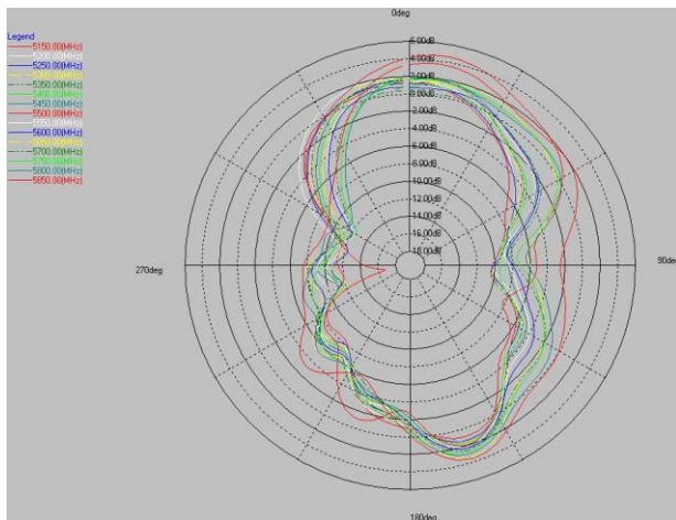
5G theta=90deg
