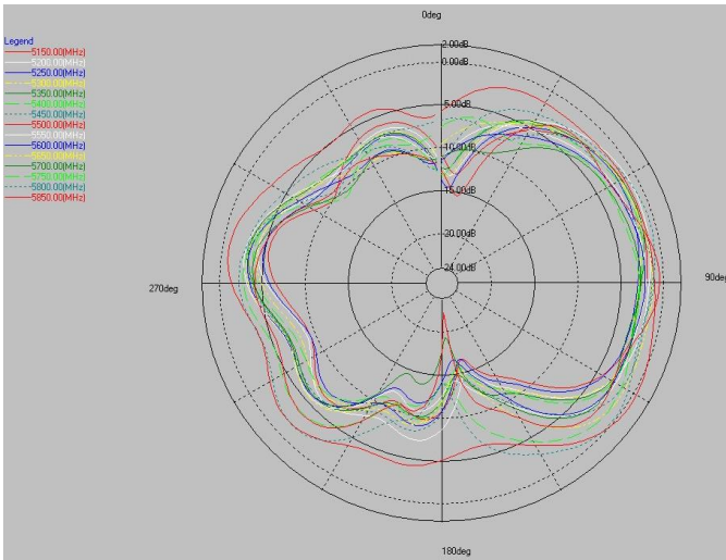
5G theta=90deg
