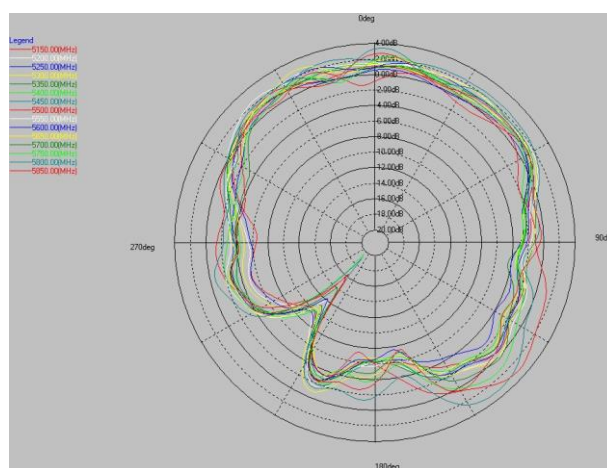
5G phi=90deg
