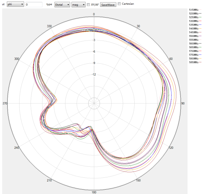
5G phi=0deg
