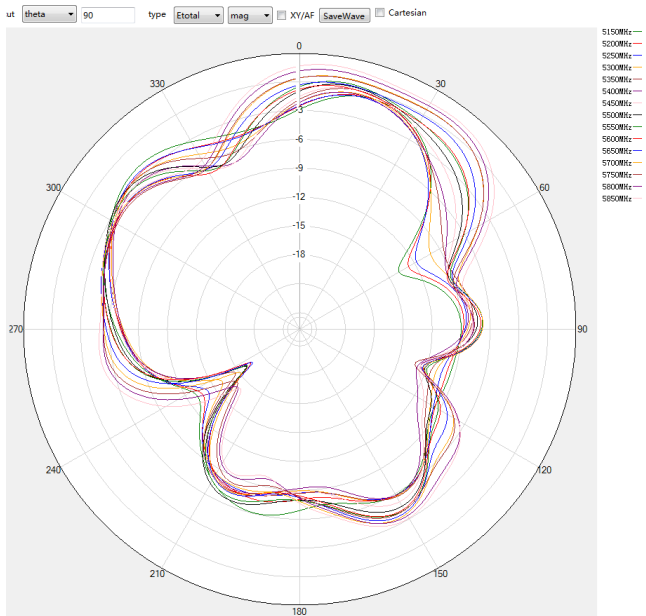
5G theta=90deg
