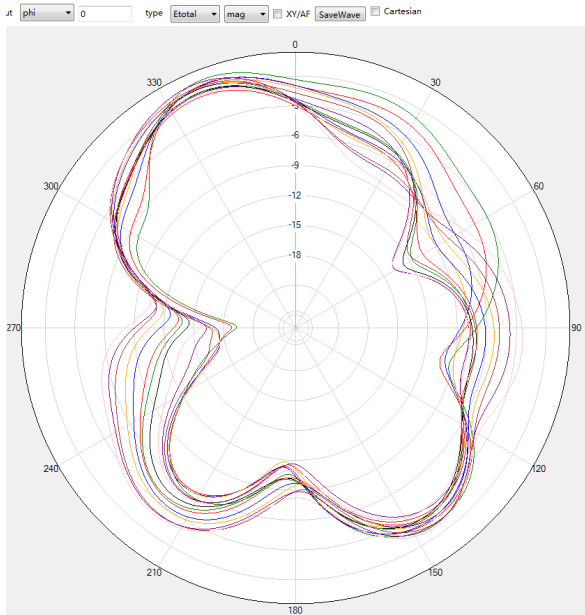
5G phi=0deg
