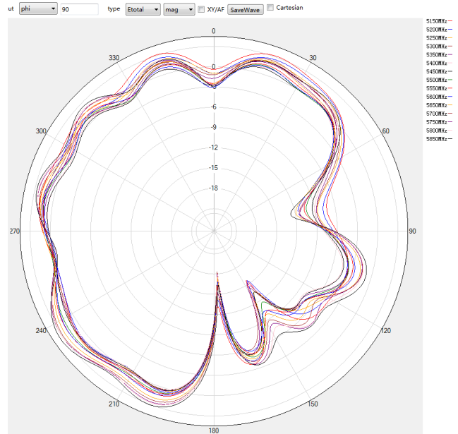
5G phi=90deg
