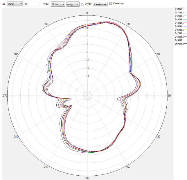
2.4G theta=90deg
