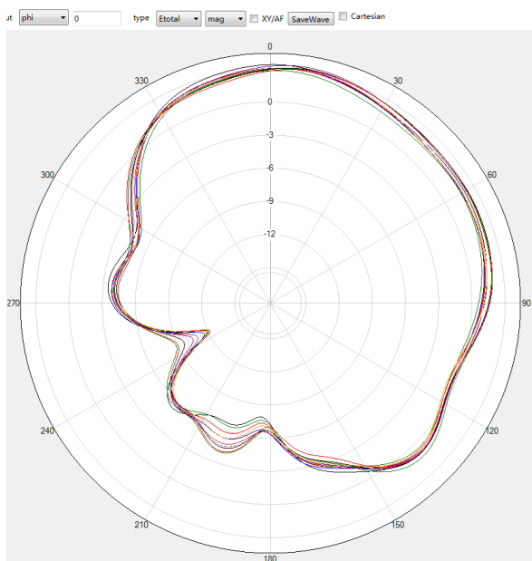
2.4G phi=0deg
