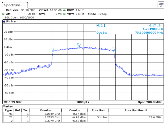
802.11ac80_5290MHz_Chain 2 75.600MHz
