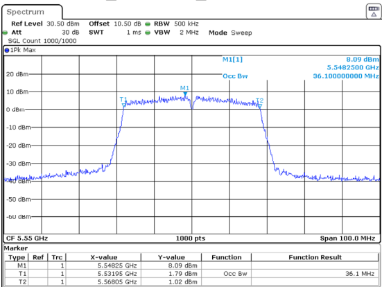
802.11ac40_5550MHz_Chain 1 36.100MHz
