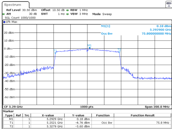
802.11ac80_5290MHz_Chain 0 75.800MHz
