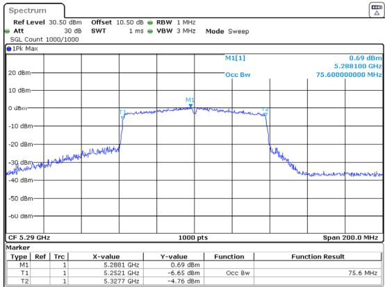
802.11ac80_5290MHz_Chain 1 75.600MHz
