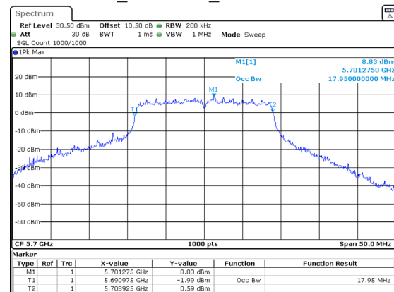
802.11ac20_5700MHz_Chain 0 17.950MHz
