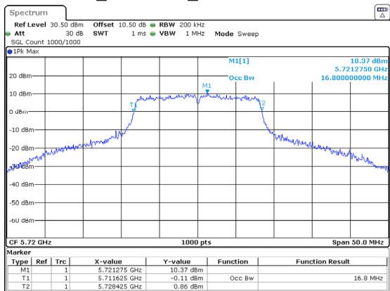
802.11a_5720MHz_Chain 0 16.800MHz
