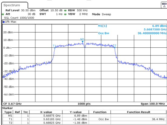
802.11ac40_5670MHz_Chain 1 36.400MHz
