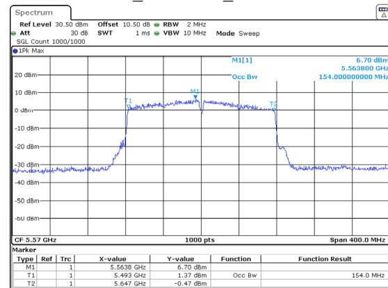
802.11ac160_5570MHz_Chain 1 154MHz
