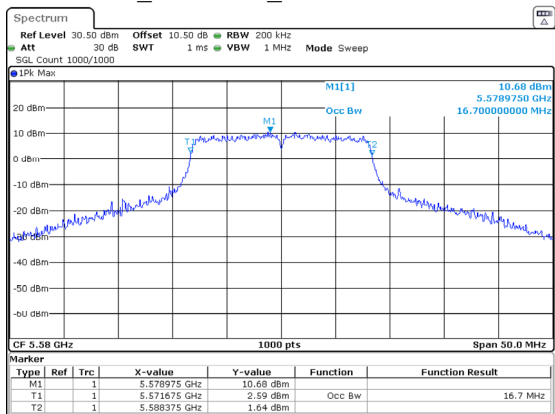
802.11a_5580MHz_Chain 1 16.700MHz
