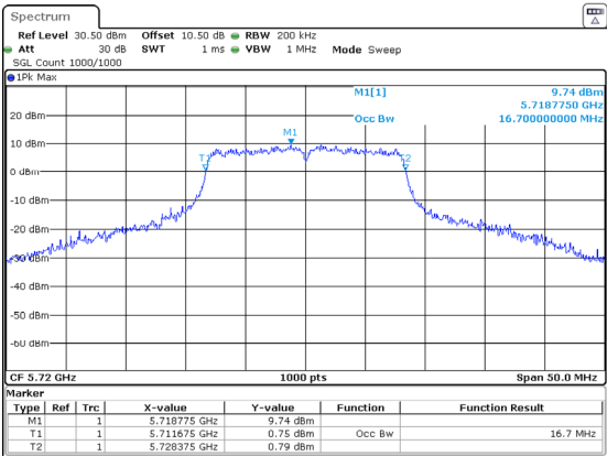
802.11a_5720MHz_Chain 1 16.700MHz
