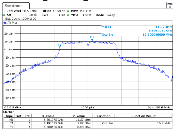
802.11a_5500MHz_Chain 1 16.800MHz
