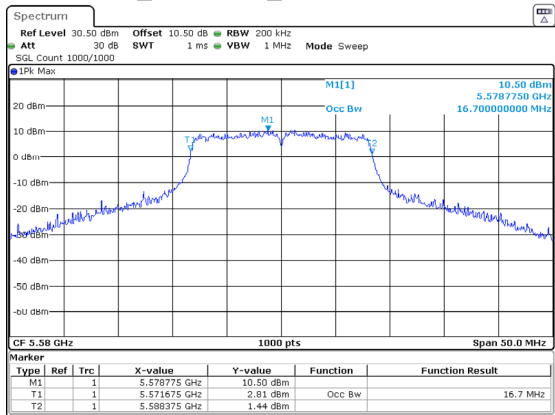
802.11a_5580MHz_Chain 0 16.700MHz
