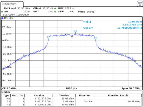
802.11a_5500MHz_Chain 2 16.750MHz
