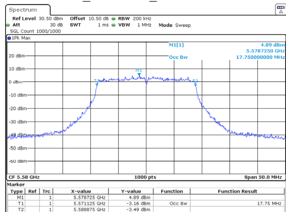
802.11ac20_5580MHz_Chain 0 17.750MHz
