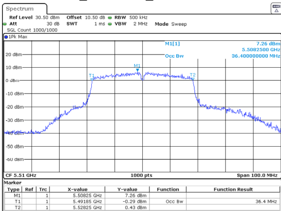
802.11ac40_5510MHz_Chain 2 36.400MHz
