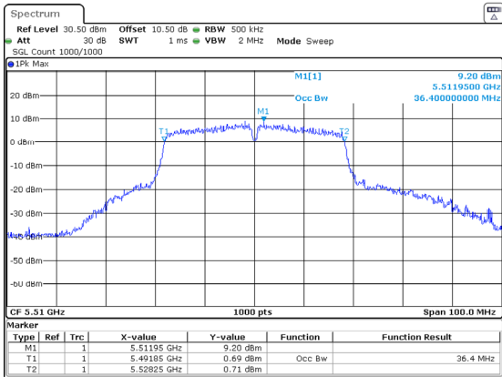
802.11ac40_5510MHz_Chain 1 36.400MHz
