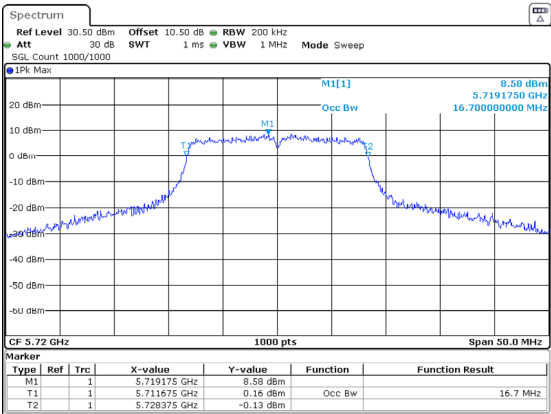
802.11a_5720MHz_Chain 2 16.700MHz
