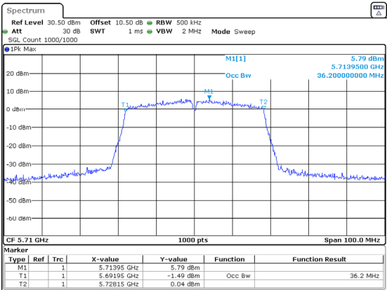
802.11ac40_5710MHz_Chain 0 36.200MHz
