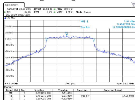
802.11ac20_5500MHz_Chain 0 17.950MHz
