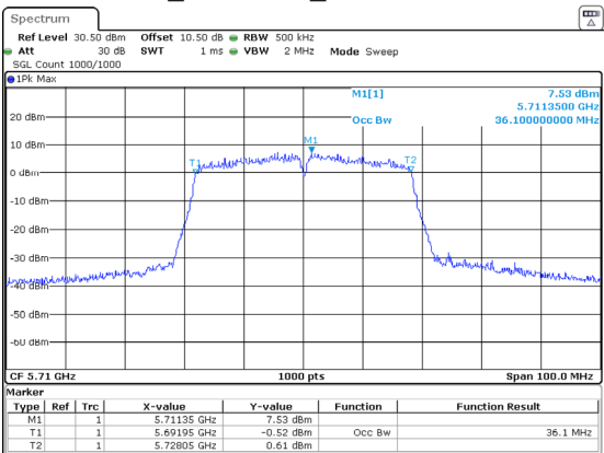
802.11ac40_5710MHz_Chain 1 36.100MHz
