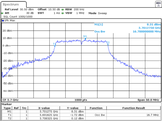
802.11a_5700MHz_Chain 2 16.700MHz
