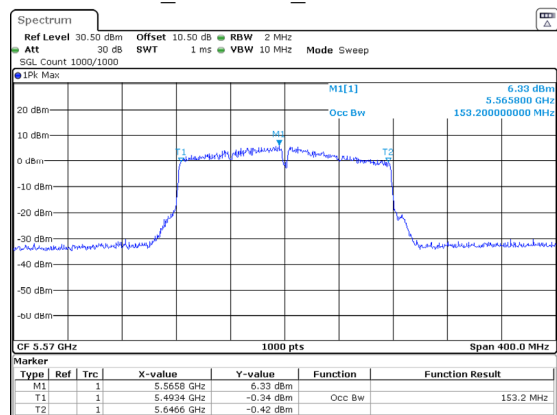
802.11ac160_5570MHz_Chain 2 153.200MHz
