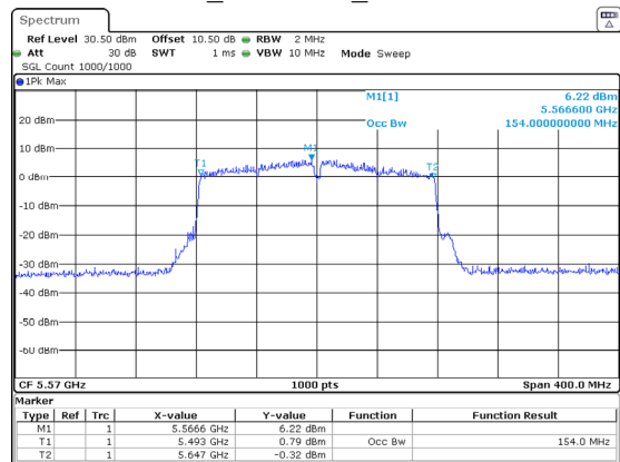
802.11ac160_5570MHz_Chain 0 154MHz
