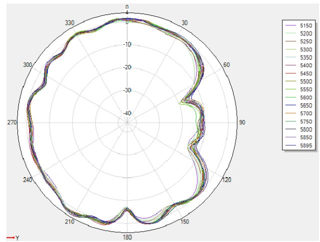
5G phi=90deg
