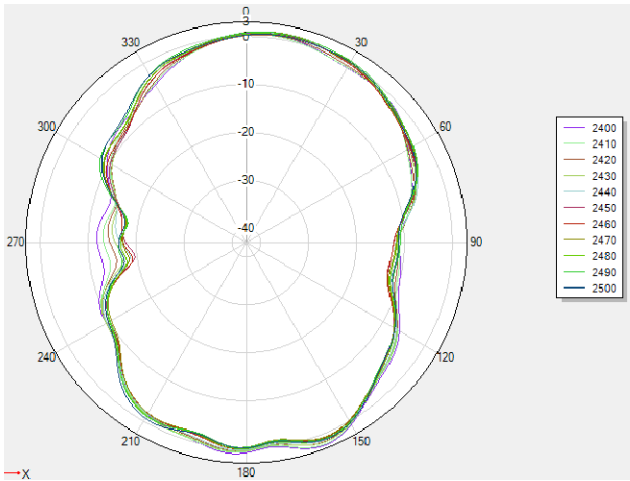
2.4G phi=0deg
