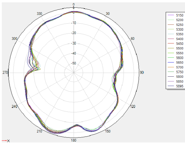
5G phi=0deg
