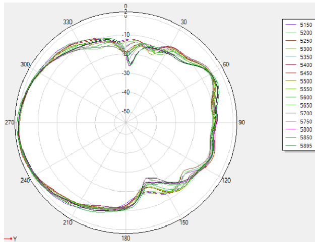
5G theta=90deg
