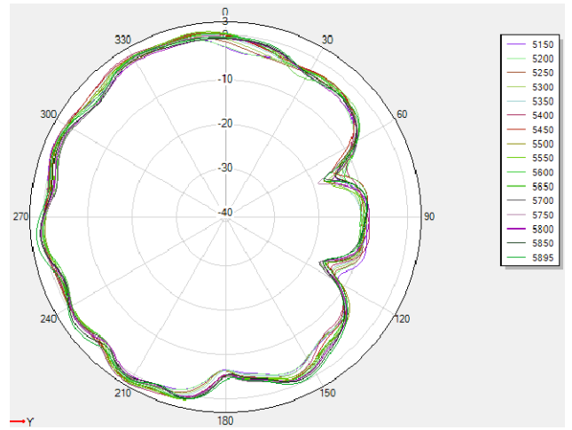
5G phi=90deg
