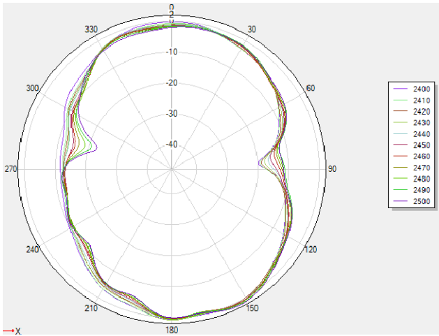
2.4G phi=0deg
