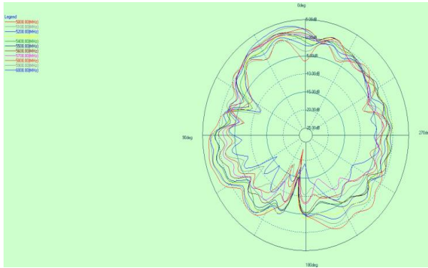
5G theta=90deg
