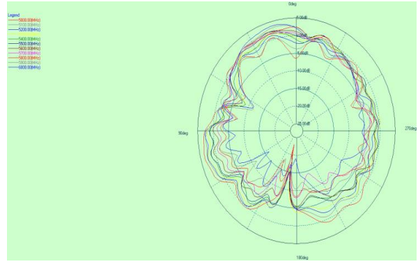
5G phi=90deg
