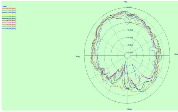
5G phi=0deg
