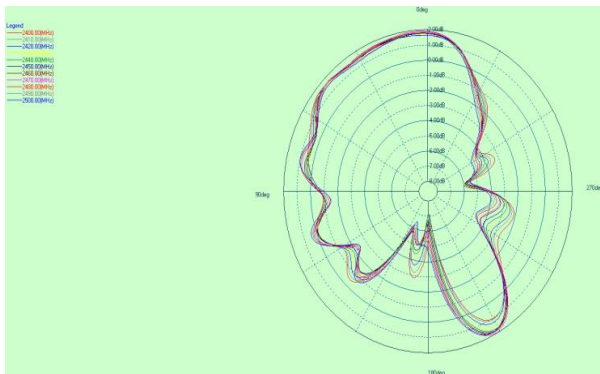
2.4G phi=0deg
