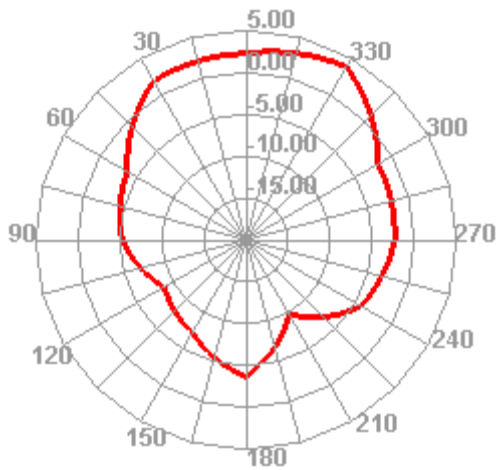
5G \theta=90^\circ
