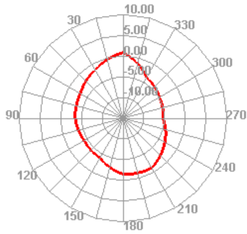
2.4G \theta=90^\circ
