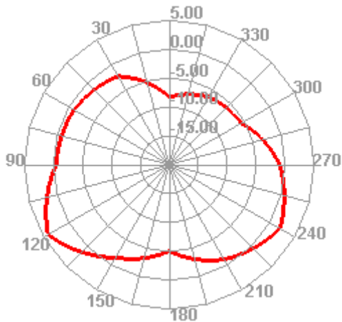
2.4G phi=0deg
