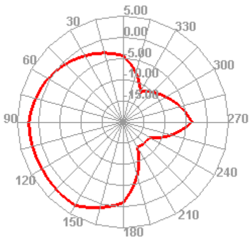
5G \phi=0^\circ
