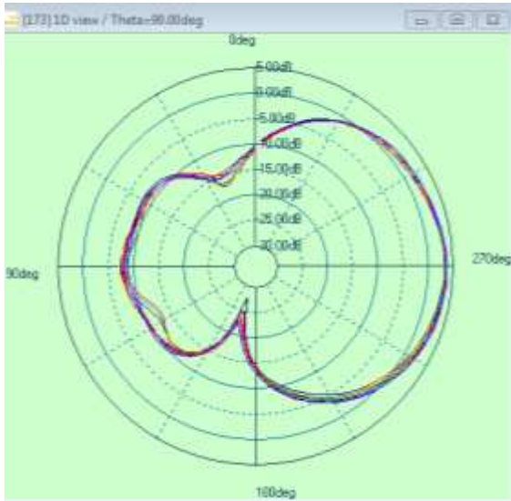
2.4G theta=90deg
