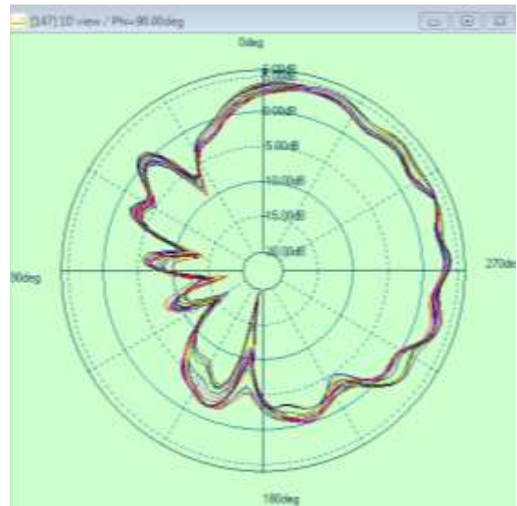
5G phi=90deg
