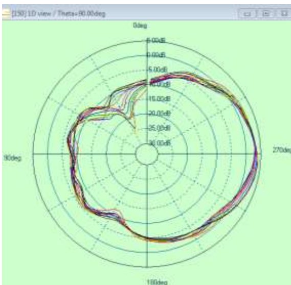
5G theta=90deg
