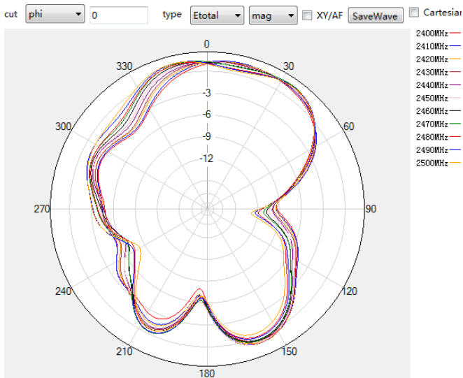
2.4G phi=0deg
