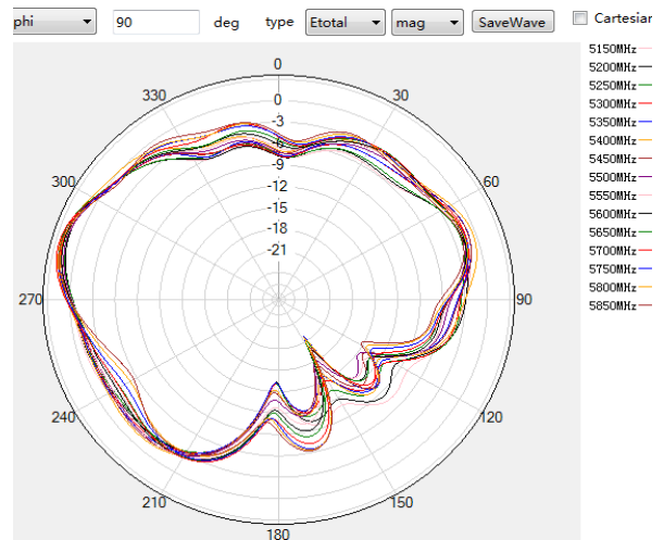
5G phi=90deg
