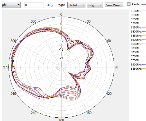
5G phi=0deg
