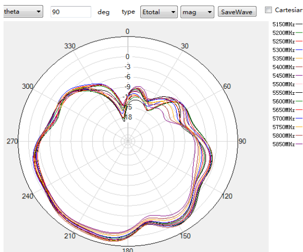
5G theta=90deg
