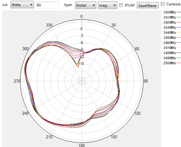
2.4G theta=90deg
