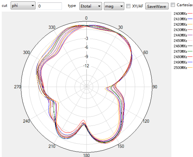
2.4G phi=0deg
