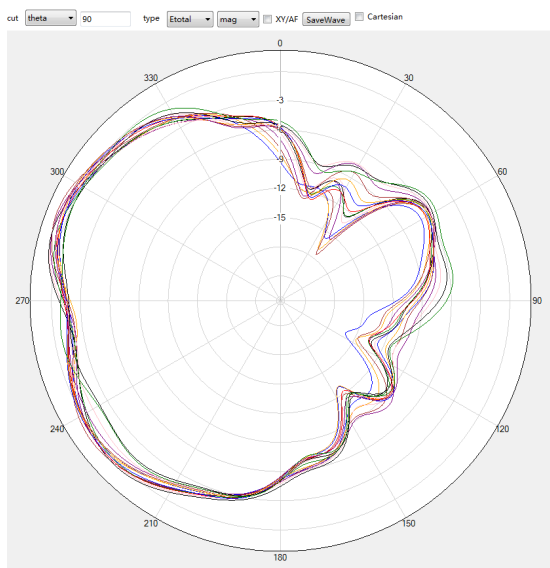
5G theta=90deg
