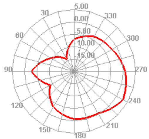
5G phi=90deg
