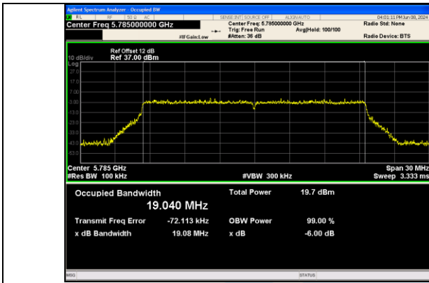
IEEE 802.11ax_Channel 157_20MHz_Antenna 0_RU&Index SU
