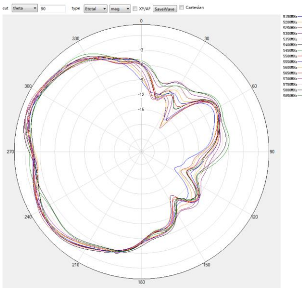
5G theta=90deg
