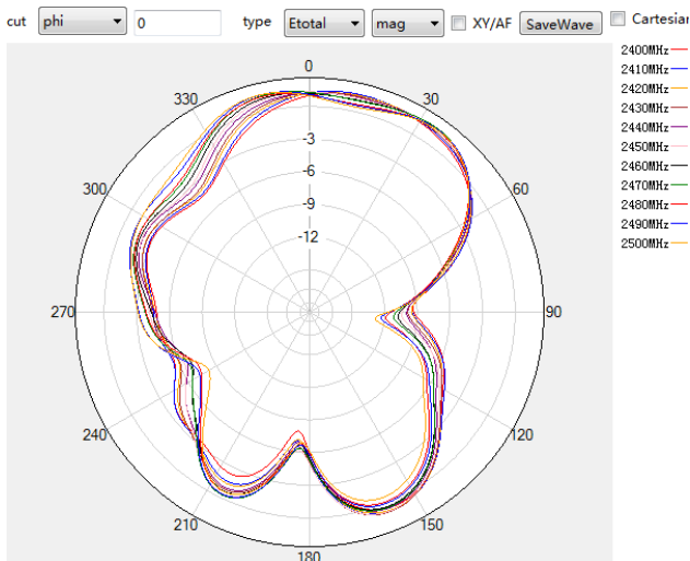
2.4G phi=0deg
