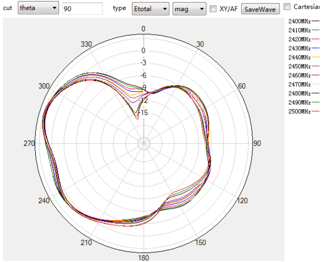
2.4G theta=90deg
