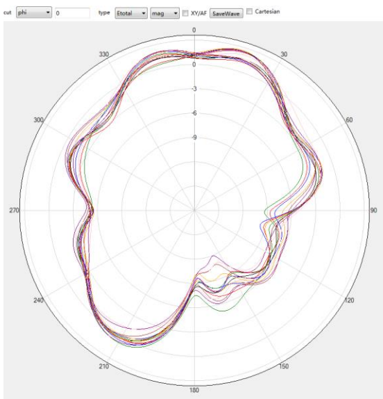
5G phi=0deg
