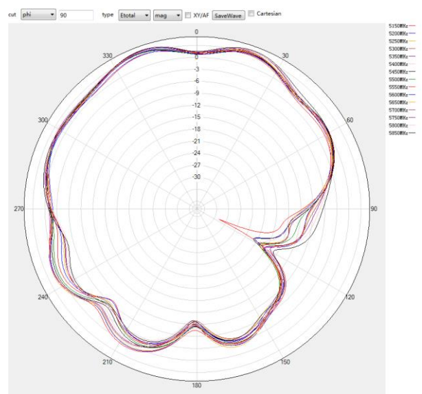
5G phi=90deg
