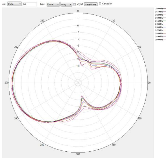
2.4G theta=90deg
