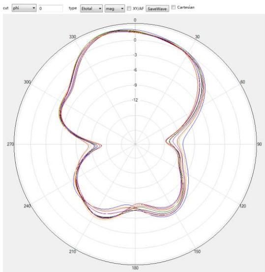
2.4G phi=0deg
