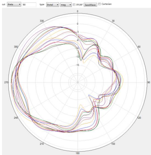
5G theta=90deg
