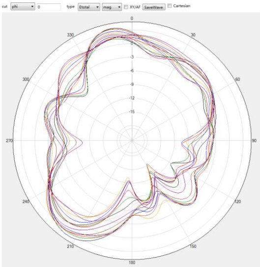
5G phi=0deg
