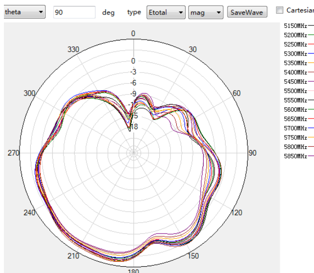
5G theta=90deg
