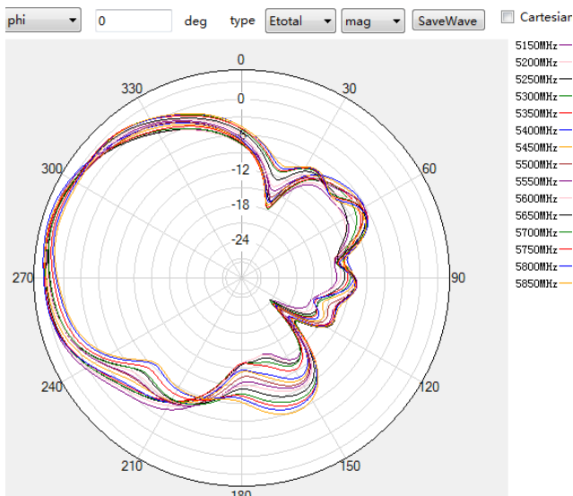
5G phi=0deg
