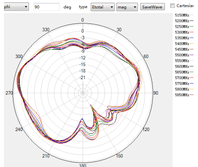
5G phi=90deg
