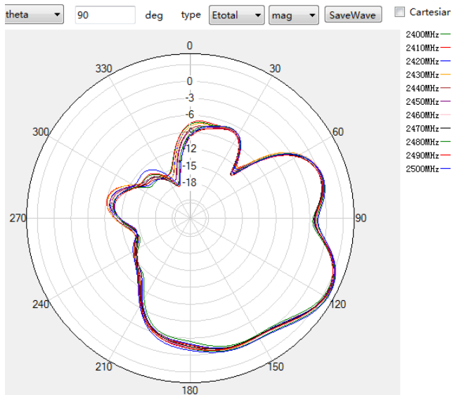
2.4G theta=90deg
