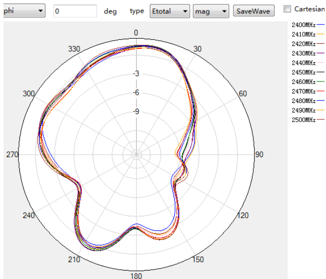
2.4G phi=0deg
