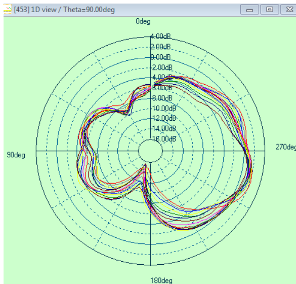
5G theta=90deg
