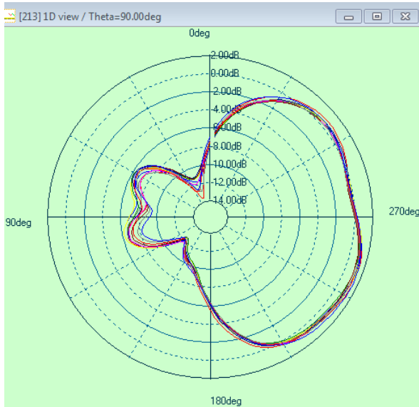
2.4G theta=90deg
