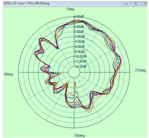
5G phi=90deg
