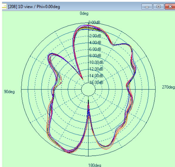
2.4G phi=0deg
