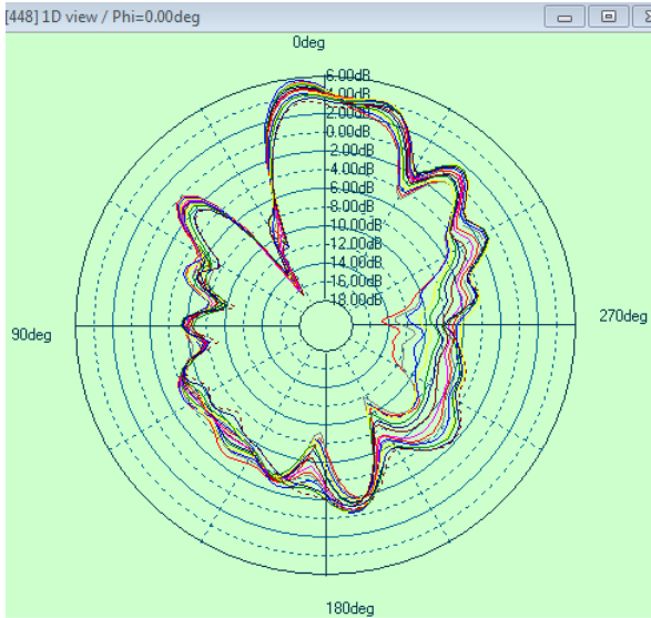
5G phi=0deg
