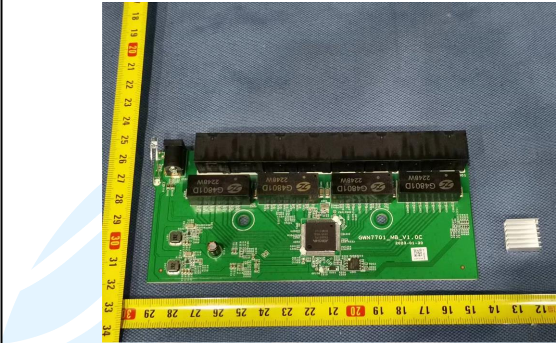
EUT Photo
