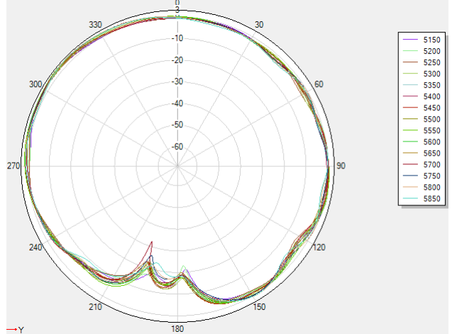
5G \phi=90^\circ
