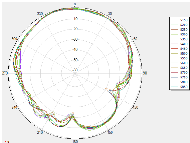
5G \phi=0^\circ
