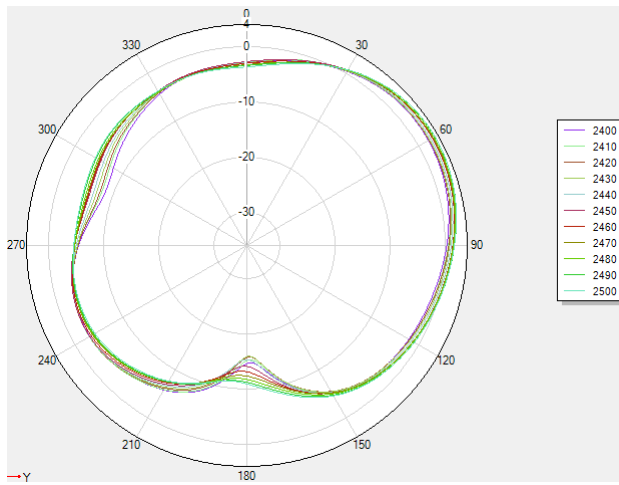
2.4G \theta=90^\circ
