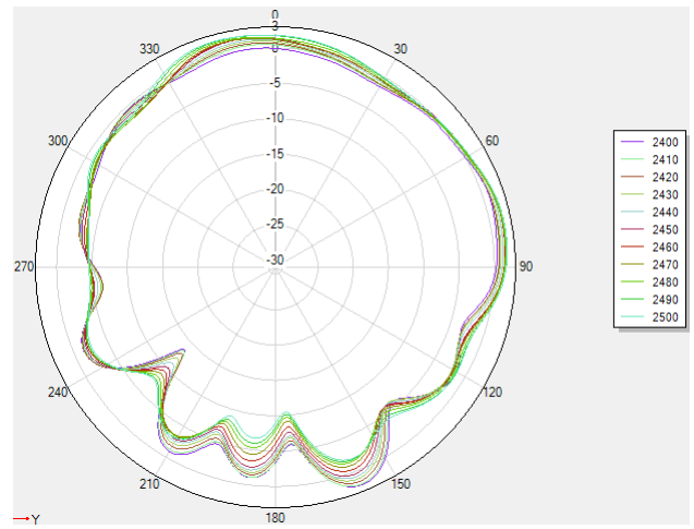
2.4G \phi=90^\circ
