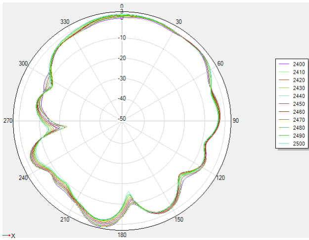
2.4G \phi=0^\circ
