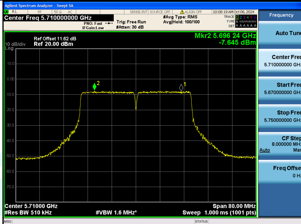
11N40SISO-Ant1-5710_UNII-3-PASS
