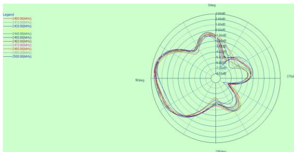
2.4G theta=90deg
