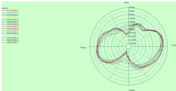
5G theta=90deg
