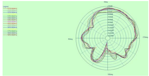
5G phi=90deg
