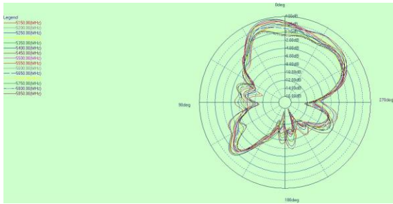
5G phi=0deg
