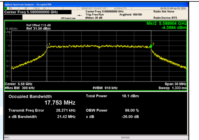
IEEE 802.11ac_Channel 116_20MHz_Antenna 1
