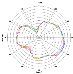
2.4G phi=0deg
