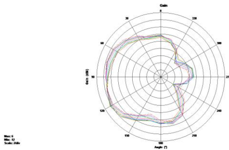
2.4G theta=90deg
