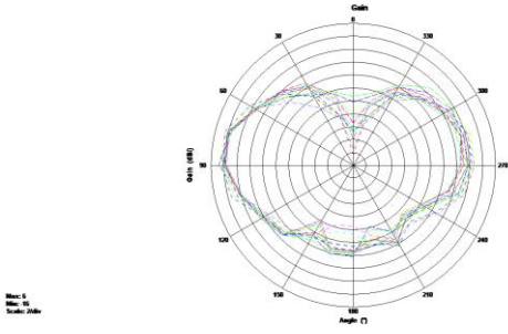
5G phi=0deg
