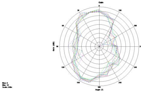
5G theta=90deg
