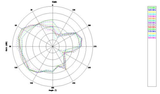
5G phi=90deg
