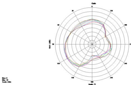
2.4G theta=90deg
