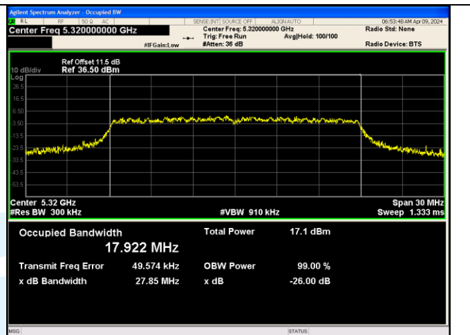
IEEE 802.11ac_Channel 64_20MHz_Antenna 1
