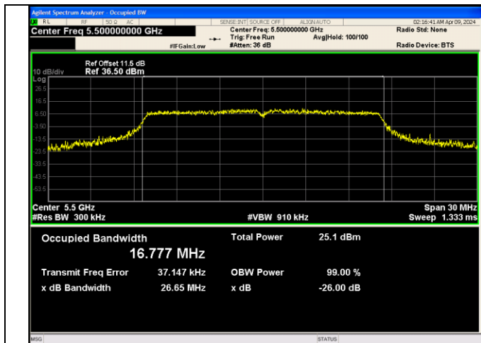
IEEE 802.11a_Channel 100_20MHz_Antenna 0
