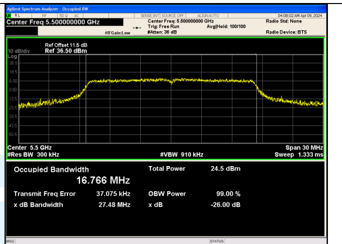
IEEE 802.11a_Channel 100_20MHz_Antenna 1
