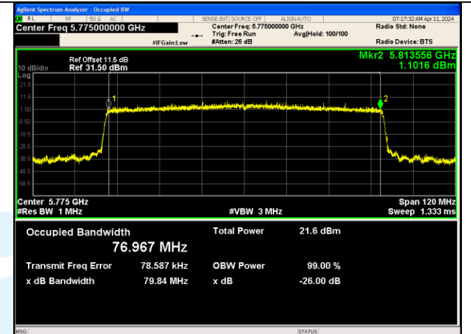
IEEE 802.11ax_Channel 155_80MHz_Antenna 1_RU&Index SU
