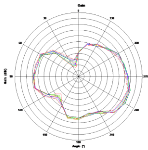
2.4G phi=0deg
