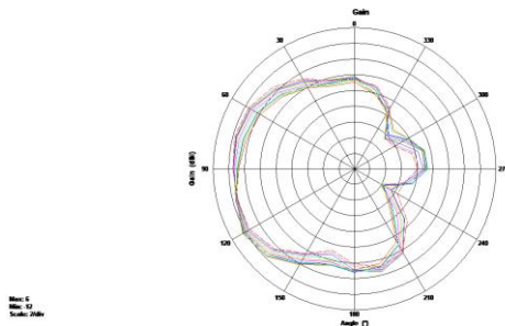
2.4G theta=90deg
