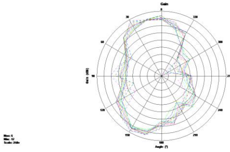
5G theta=90deg
