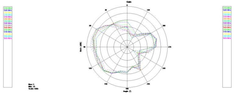
5G phi=90deg
