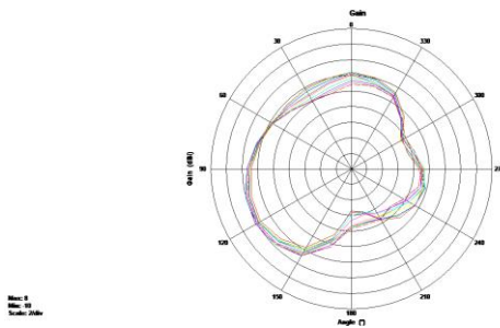
2.4G theta=90deg
