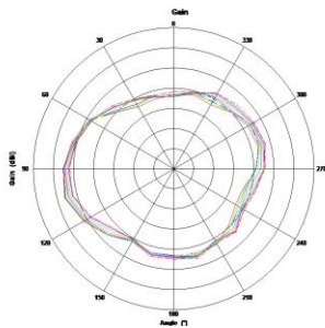
2.4G phi=0deg
