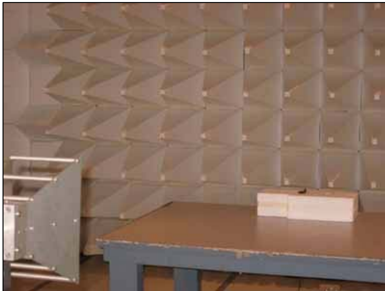
RSS 210 1-18GHz
