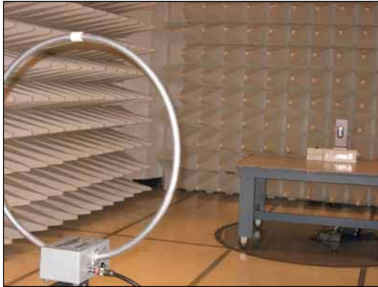
15.249(d) 0.09-30MHz
