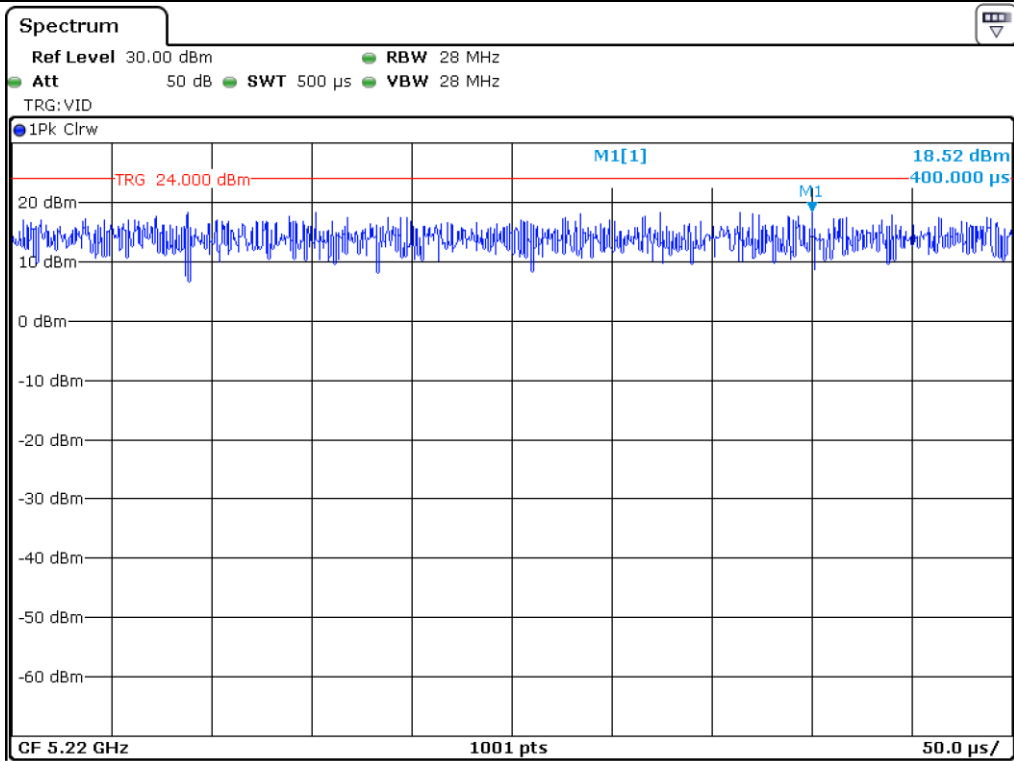
802.11 n(HT20)
