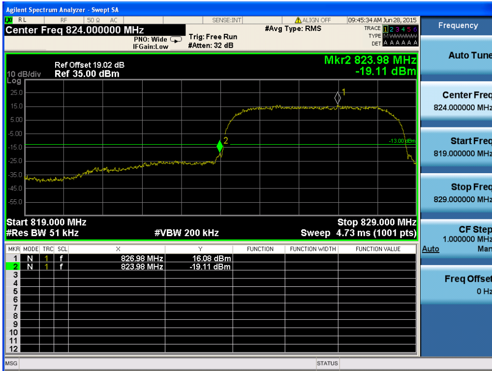
WCDMA850& Channel: 4132
