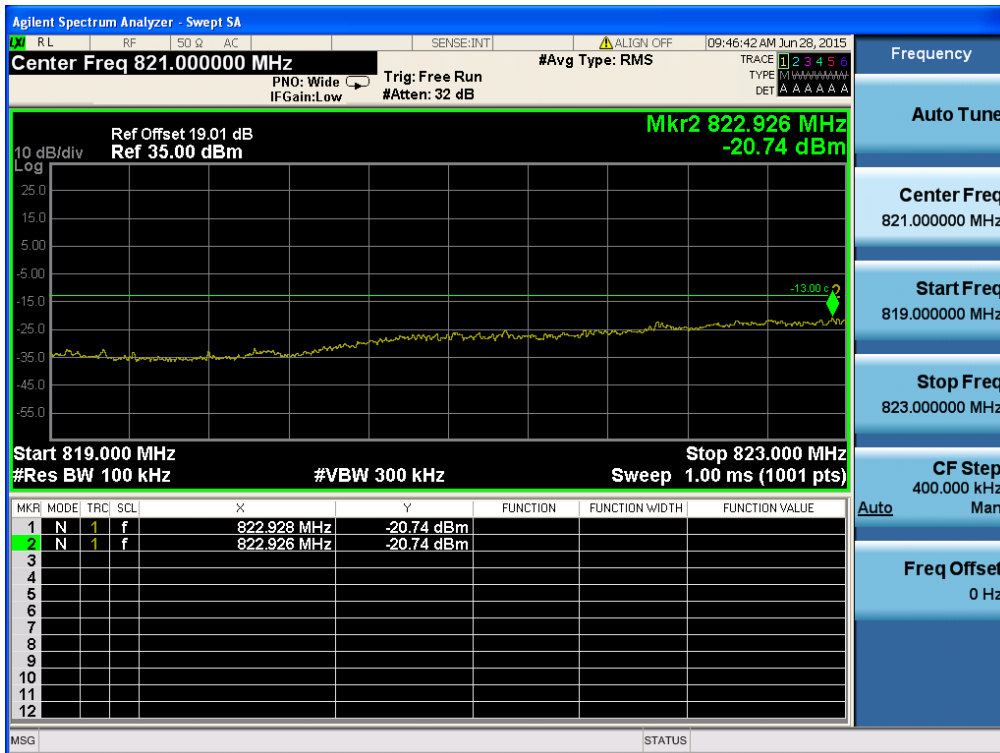
WCDMA850& Channel: 4132
