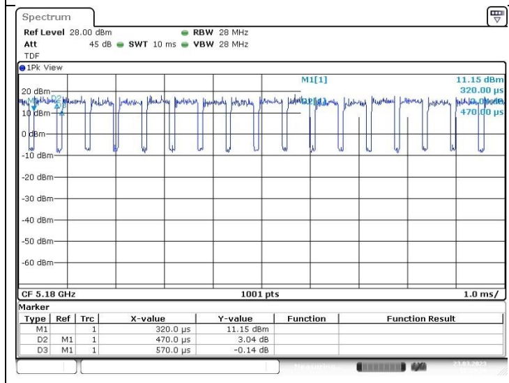
802.11ac_VHT20
